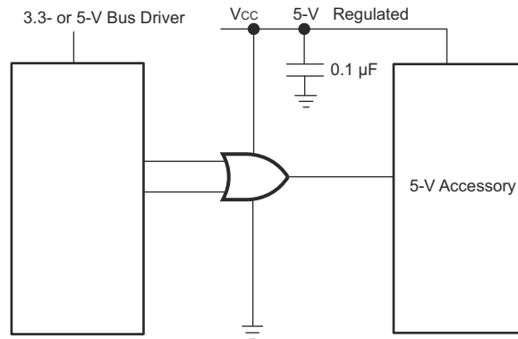
图 8-1. 单门的典型应用图
