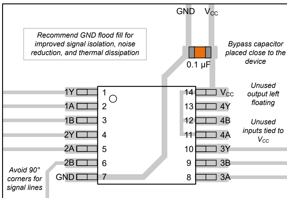
图 8-3. 示例布局 SN54SC4T02-SEP
