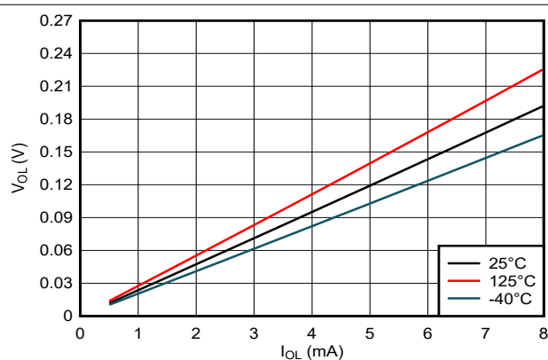
图 6-10. 低电平状态下输出电压与电流间的关系；2.5V 电源
