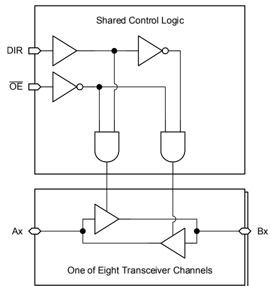
简化逻辑图
