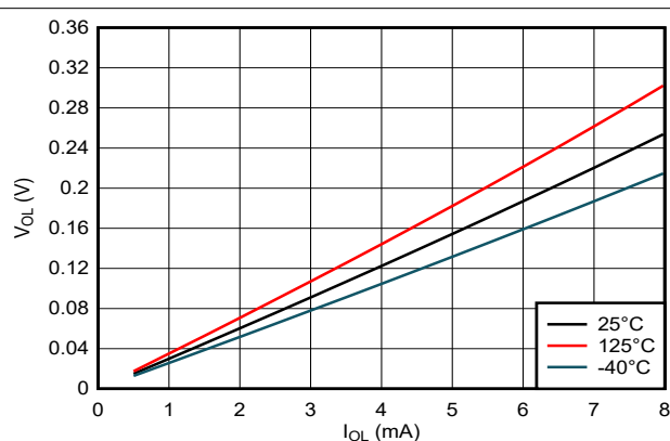
图 6-12. 低电平状态下输出电压与电流间的关系；1.8V 电源
