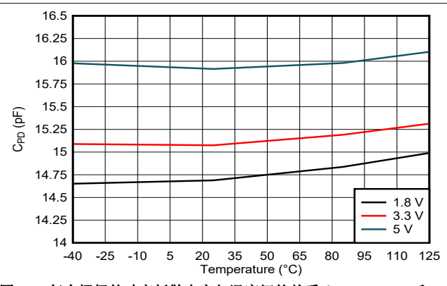
图 6-4. 每个栅极的功率耗散电容与温度间的关系 (1.8V、3.3V 和 5V 电源)
