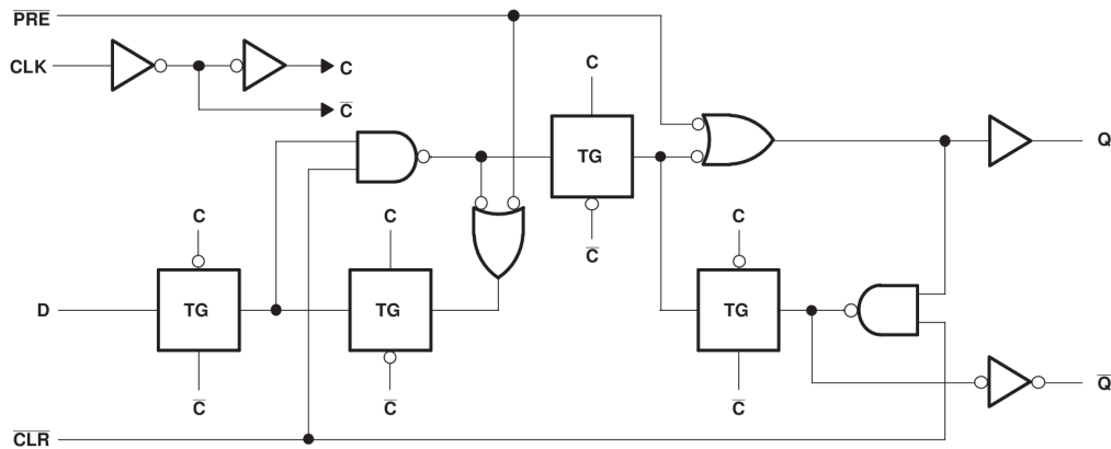
展示各触发器的逻辑图 (正逻辑)
