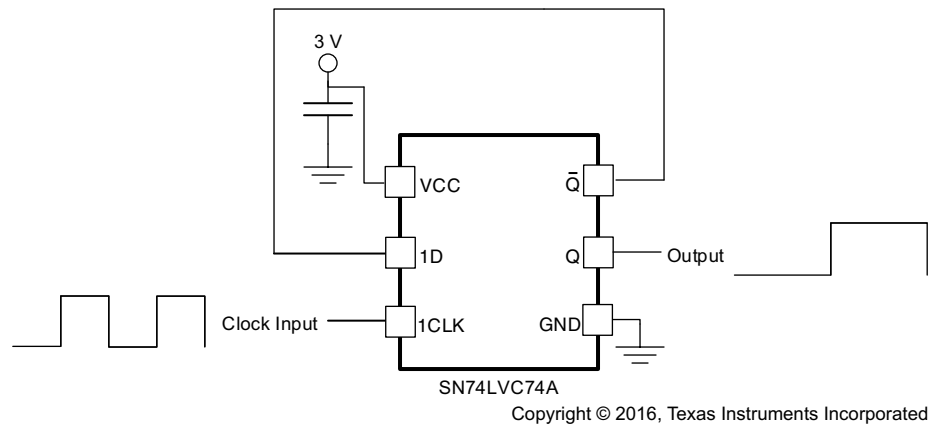
图 8-1. 分频器
