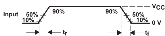
图 6-3. 输入上升和下降时间
