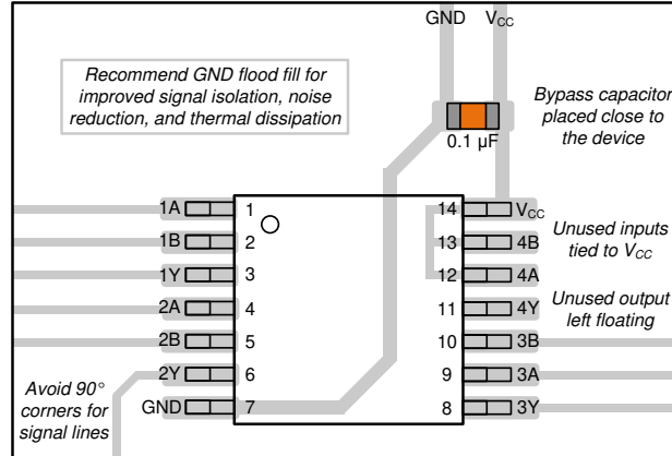
图 7-1. SNx4AC32 的布局示例
