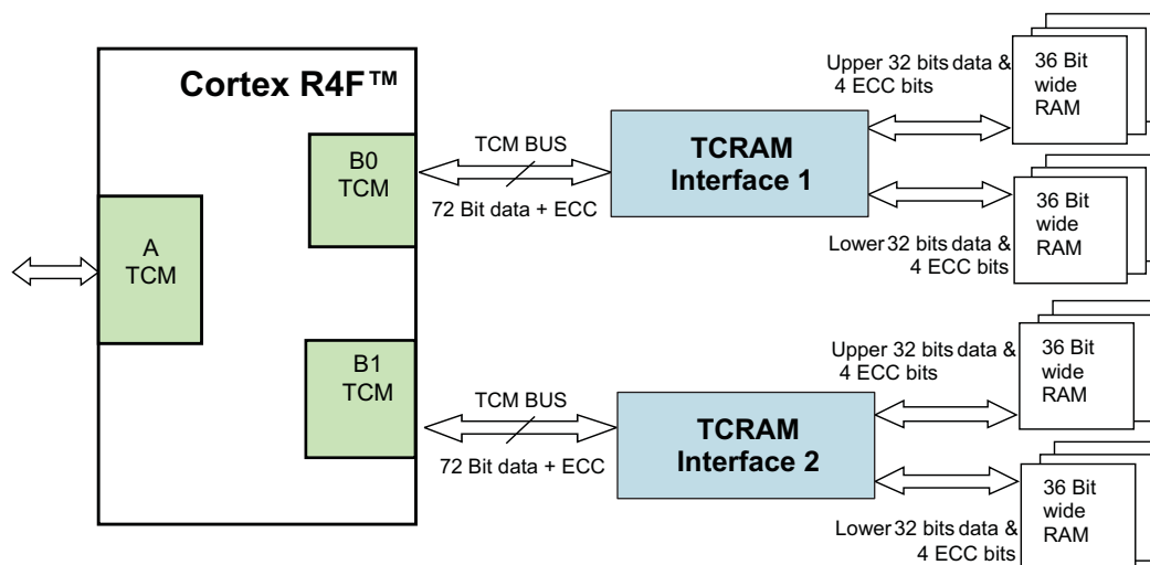
图 5-11. TCRAM 方框图
