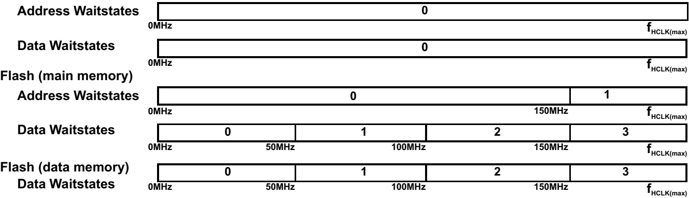
图 4-1. 等待状态机制
