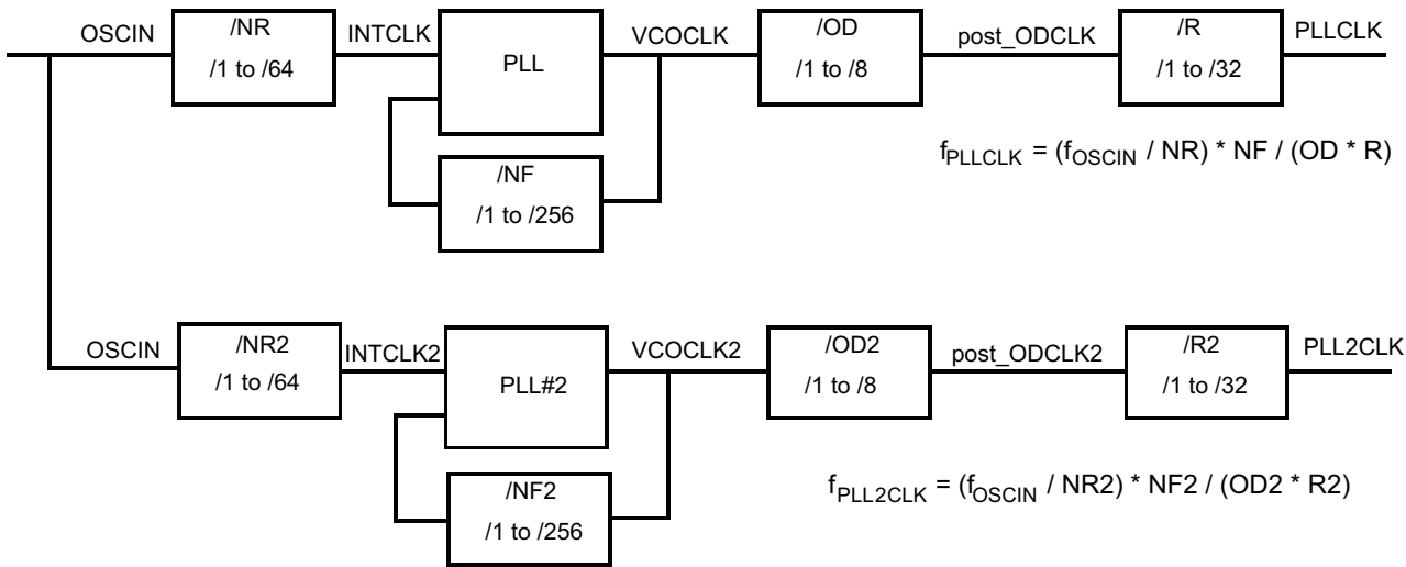
图 5-6. PLLx 方框图
