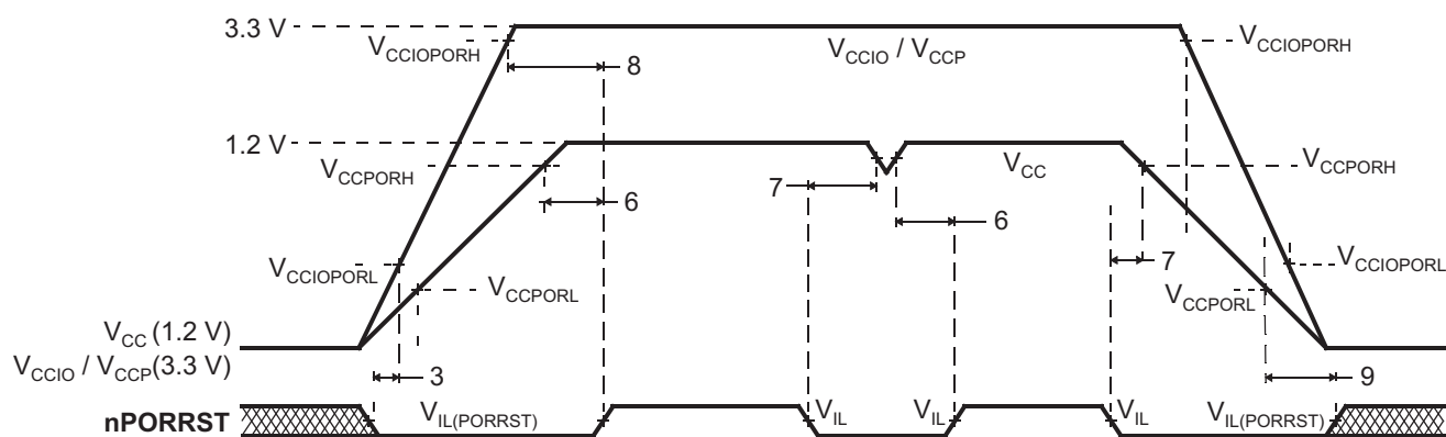
图 5-1. nPORRST 时序图
