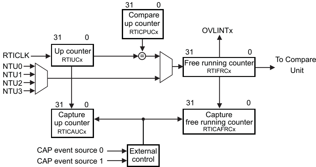
图 5-18. 计数器块图
