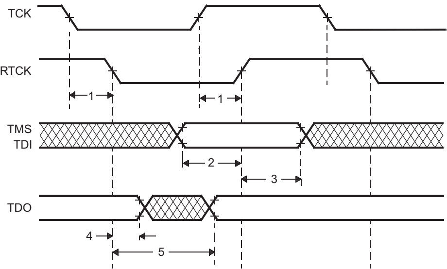
图 5-21. JTAG 时序
