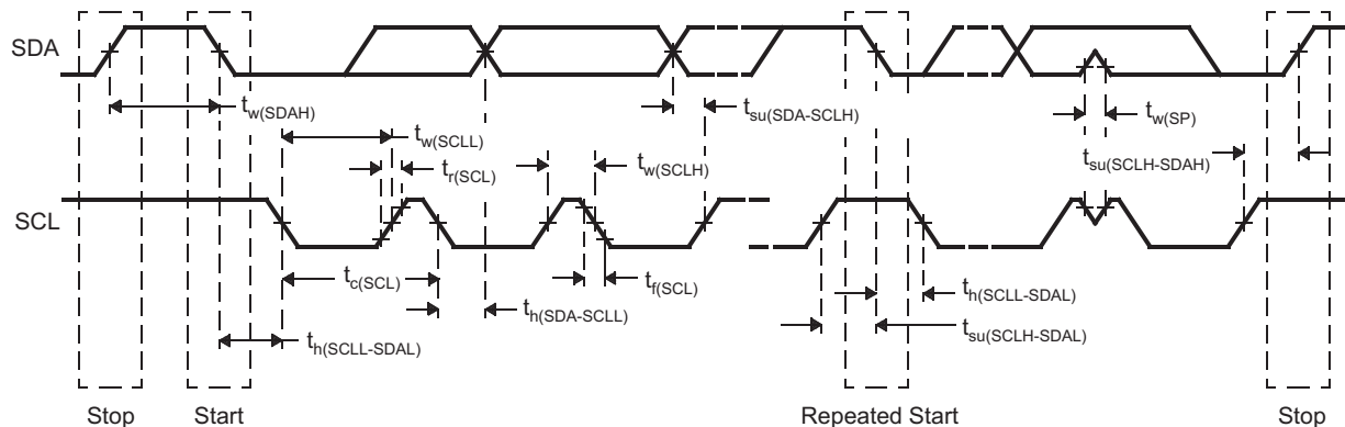
图 6-13. I2C 时序
