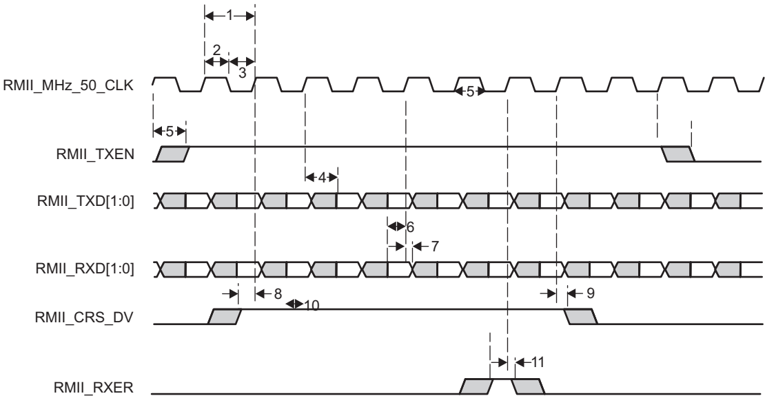
图 6-24. RMII 时序图
