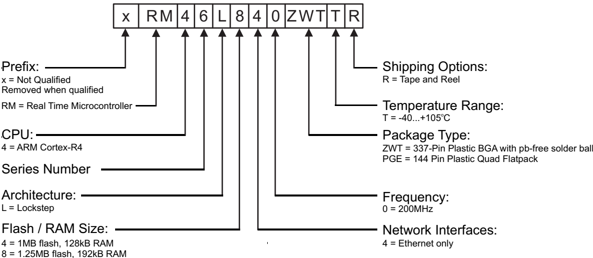
图 7-1. RM46Lx40 器件编号惯例
