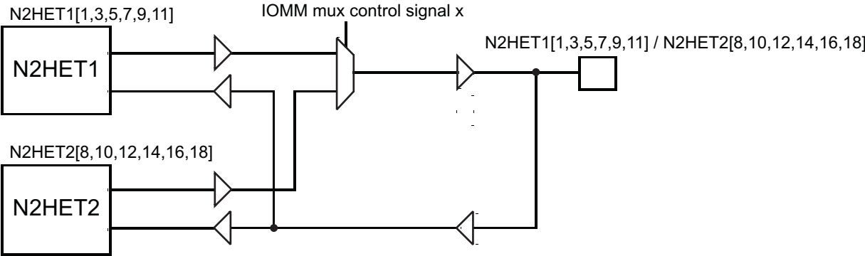
图 6-12. N2HET 监视
