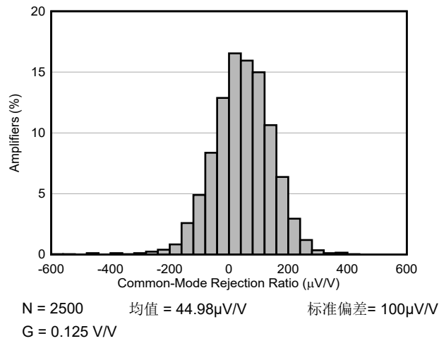
图 7-23. CMRR 分布
