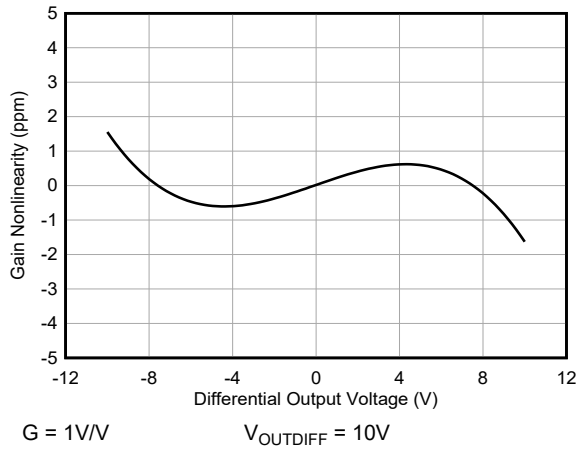
图 7-33. 增益非线性
