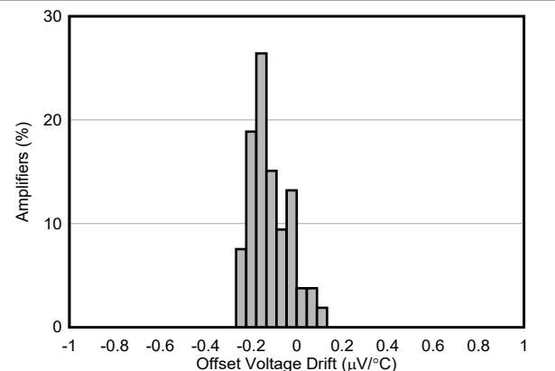
图 7-2. 失调电压漂移 (RTI) 的分布
