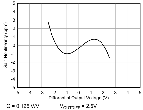
图 7-34. 增益非线性
