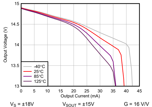
图 7-48. 正输出电压与输出电流间的关系
