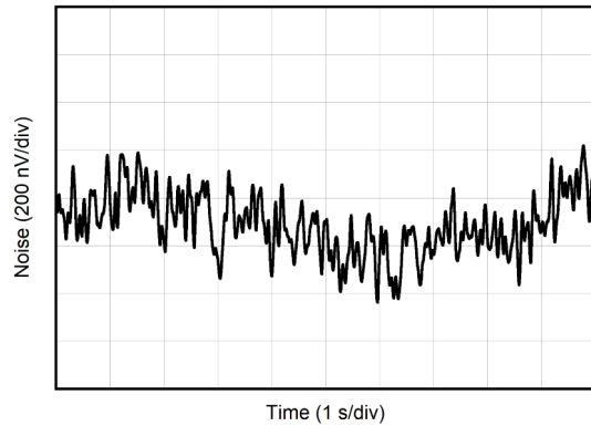
图 7-37. 0.1Hz 至 10Hz 电压噪声 (RTI)
