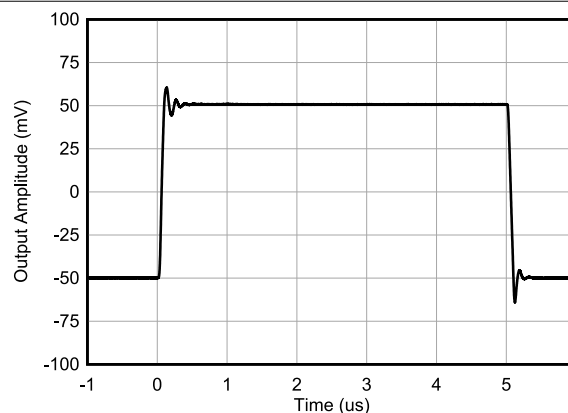
图 7-42. 小信号阶跃响应
