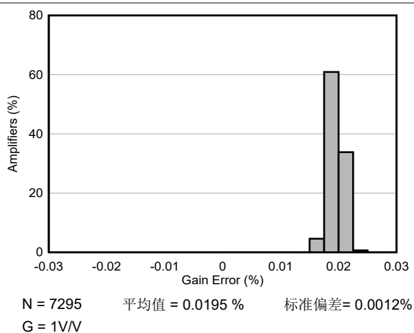
图 7-8. 差分增益误差的分布
