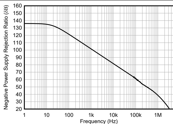
图 7-28. 负 PSRR 与频率间的关系
