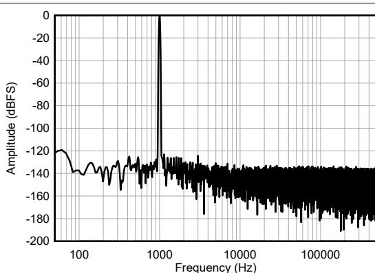
图 9-10. 使用 ADS8900B 的性能 FFT 图
