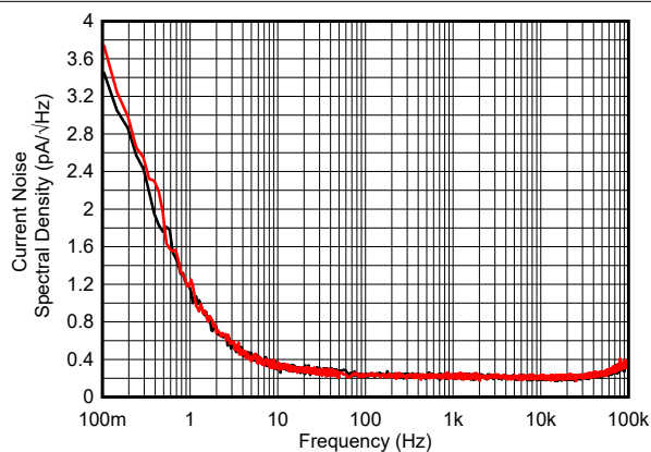
图 7-39. 电流噪声频谱密度与频率间的关系
