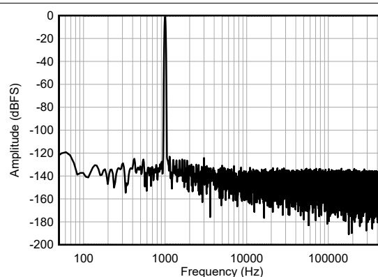
图 9-11. 使用 ADS8900B 的性能 FFT 图
