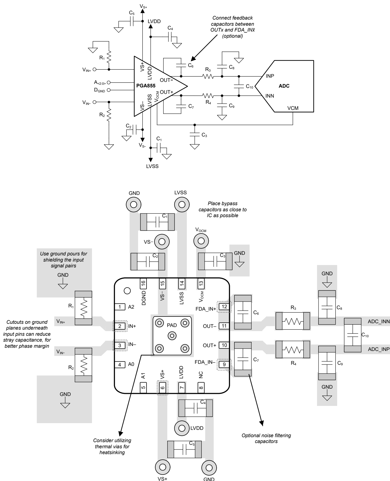
图 9-12. 原理图和相关 PCB 布局示例
