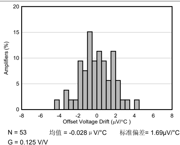
图 7-6. 失调电压漂移 (RTI) 的分布
