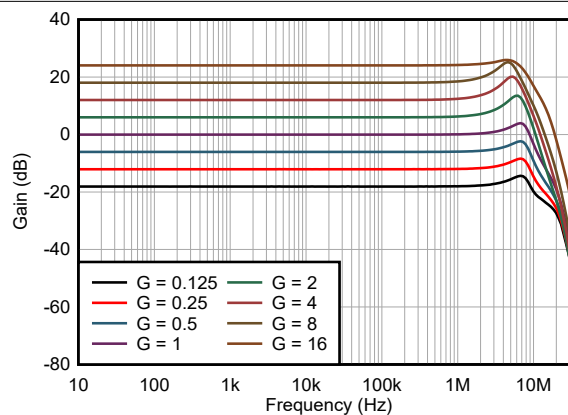
图 7-40. 增益与频率间的关系
