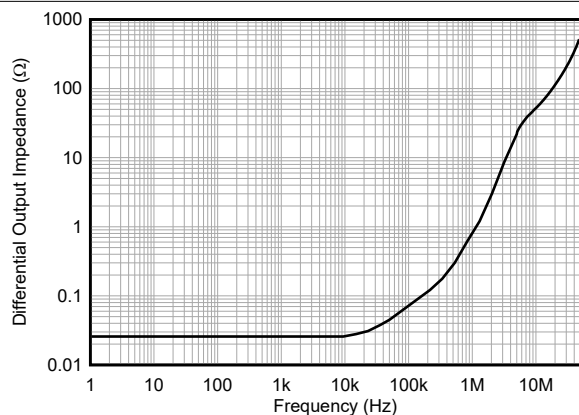
图 7-51. 闭环输出阻抗与频率间的关系
