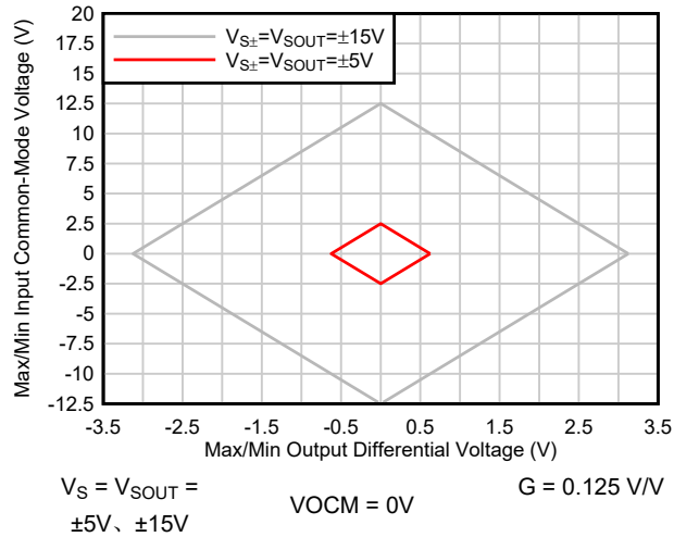
图 9-3. G = 0.125V/V 时输入共模电压与输出电压间的关系
