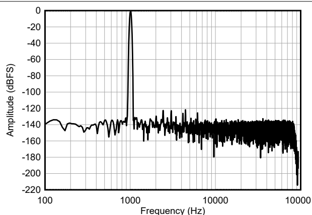
图 9-8. 使用 ADS127L11、OSR = 64、宽带滤波器时的性能 FFT 图
