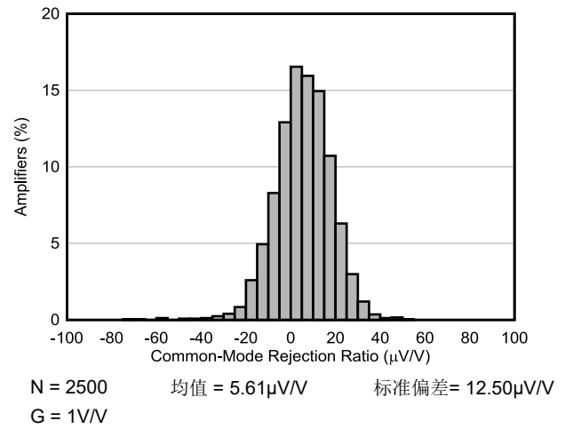
图 7-22. CMRR 分布
