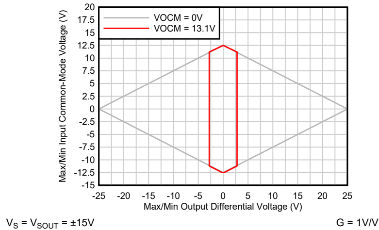
图 9-5. V_{OCM} 为最大值时输入共模电压与输出电压间的关系
