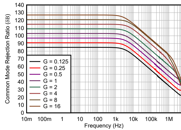
图 7-22. CMRR 分布
