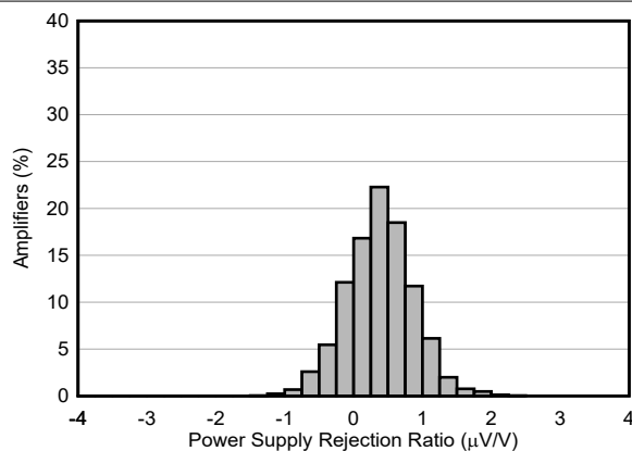
图 7-29. PSRR 分布
