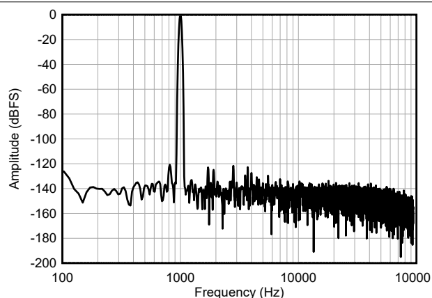
图 9-7. 使用 ADS127L11、OSR = 64、Sinc4 滤波器时的性能 FFT 图
