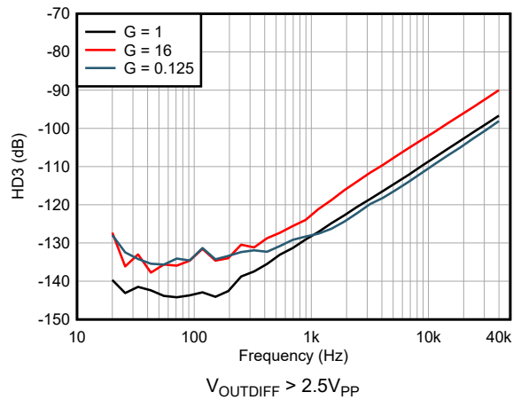
图 7-57. 三次谐波失真与频率间的关系
