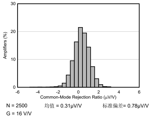
图 7-21. CMRR 分布
