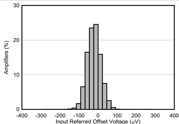
图 7-1. 失调电压 (RTI) 的分布
