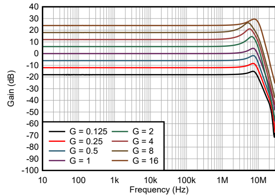
增益与频率间的关系
