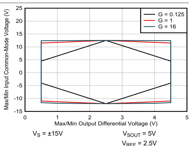
图 8-4. 输入共模电压与输出电压间的关系
