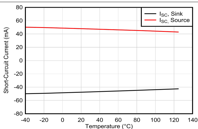
图 6-43. 输出短路电流与温度间的关系
