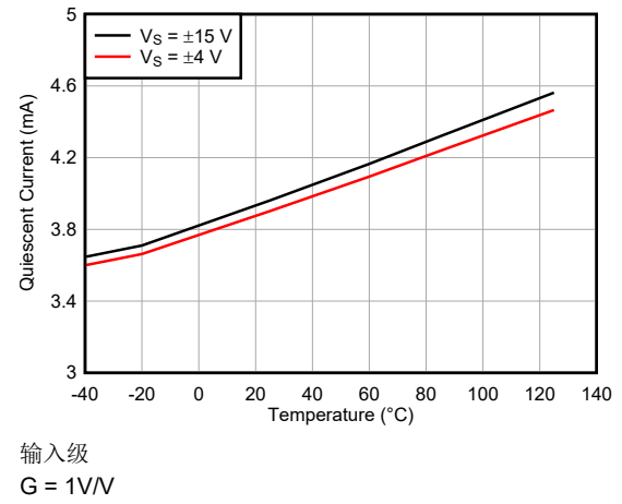
图 6-62. 静态电流与温度间的关系
