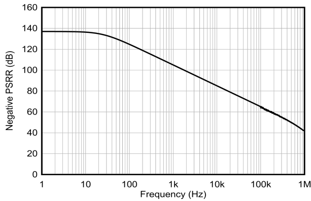
图 6-13. PSRR 分布图
