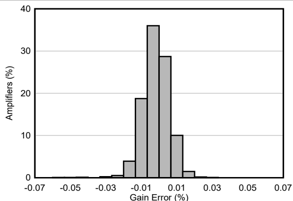
N = 1767 平均值 = -0.0017\% 标准偏差 = 0.0074\% G = 0.125\text{V/V}
