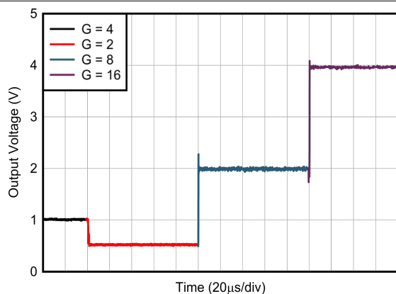
图 6-55. 增益开关瞬态响应
