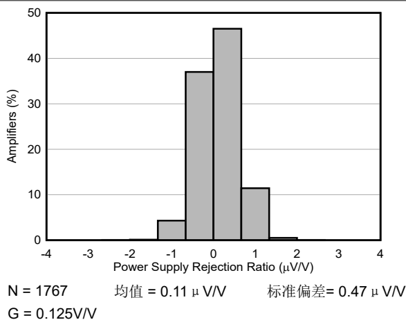
图 6-11. PSRR 分布图
