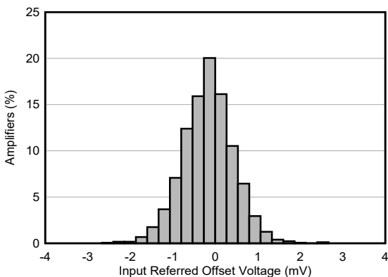
图 6-1. 失调电压 (RTI) 的分布
