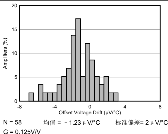
图 6-7. 失调电压漂移 (RTI) 的分布
