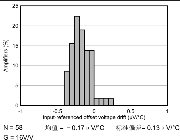
图 6-9. 失调电压漂移 (RTI) 的分布
