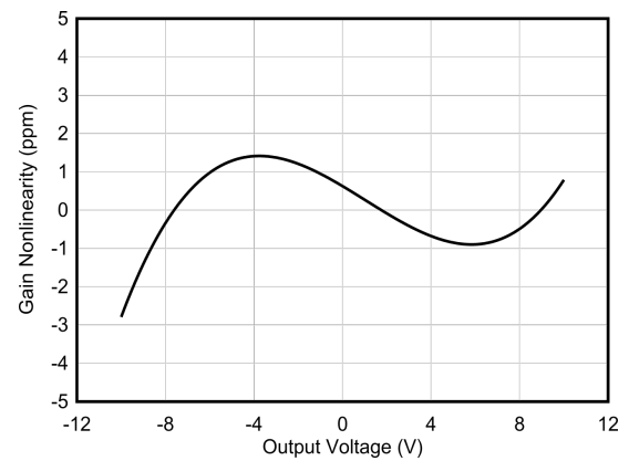
图 6-38. 增益非线性
