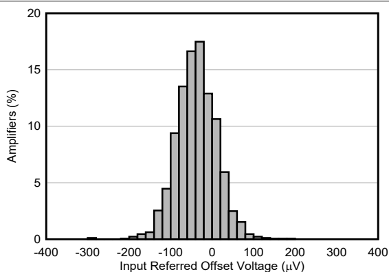
图 6-1. 失调电压 (RTI) 的分布
