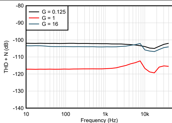
图 6-56. 总谐波失真 + 噪声与频率间的关系
