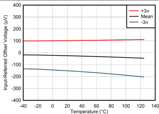
图 6-4. 失调电压 (RTI) 与温度间的关系
