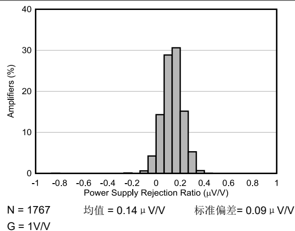
图 6-12. PSRR 分布图
