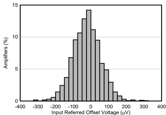
图 6-2. 失调电压 (RTI) 的分布
