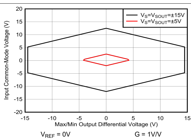
图 8-2. 输入共模电压与输出电压间的关系
