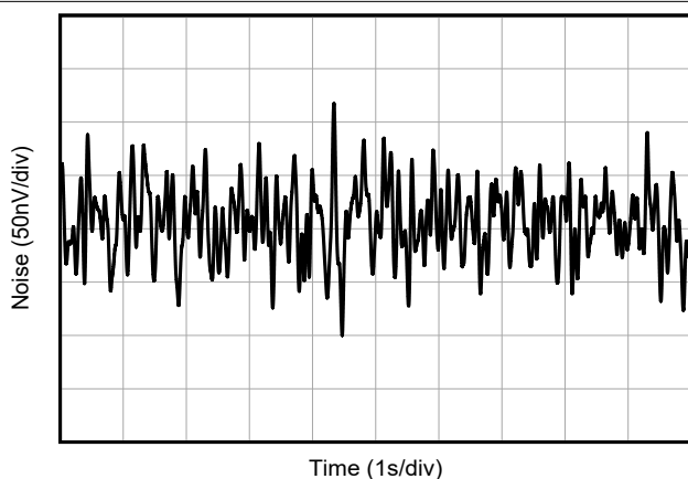
所示为典型器件 G = 16\text{V/V}
