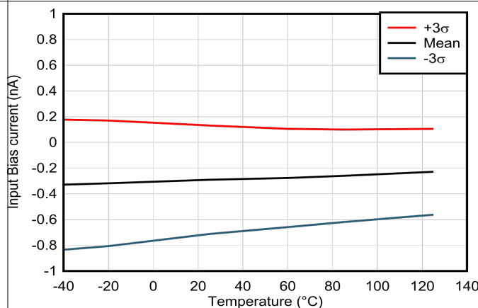
图 6-22. 输入偏置电流的分布
