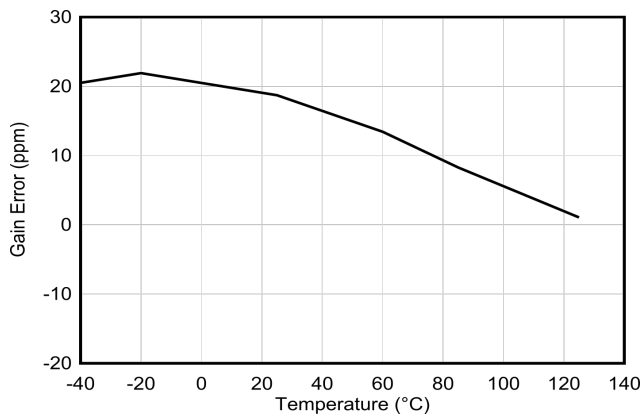
图 6-37. 增益误差与温度间的关系
