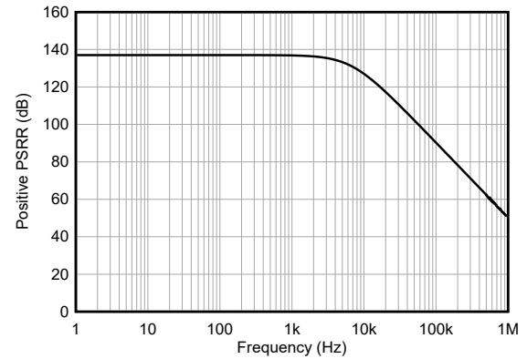
图 6-14. 正 PSRR 与频率间的关系
