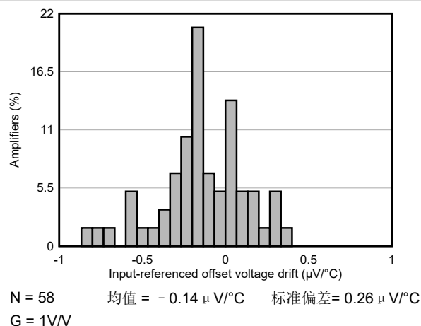
图 6-8. 失调电压漂移 (RTI) 的分布
