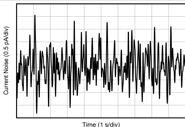
所示为典型器件 G = 1\text{V/V}
