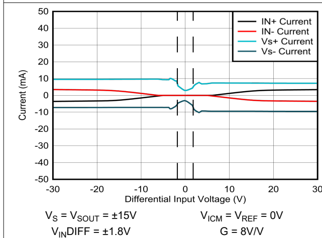
图 8-7. 电流消耗与差分输入电压间的关系
