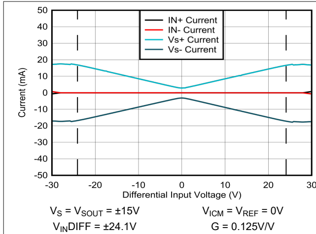
图 8-5. 电流消耗与差分输入电压间的关系
