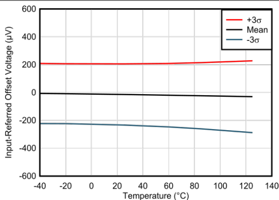
图 6-3. 失调电压 (RTI) 的分布
