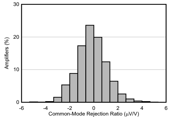
图 6-16. CMRR 分布
