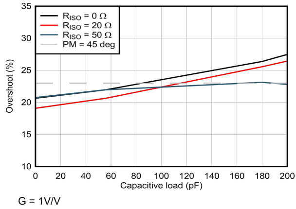
图 6-61. 过冲与容性负载间的关系
