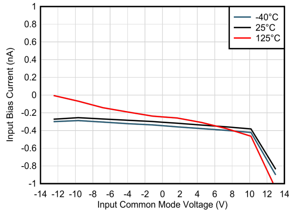
图 6-25. 输入偏置电流与 V_{\text{ICM}} 间的关系
