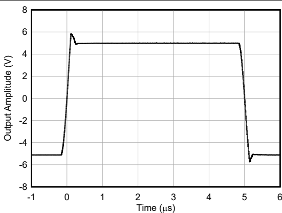
图 6-43. 过载恢复
