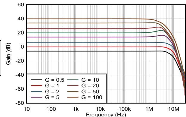
增益与频率间的关系
