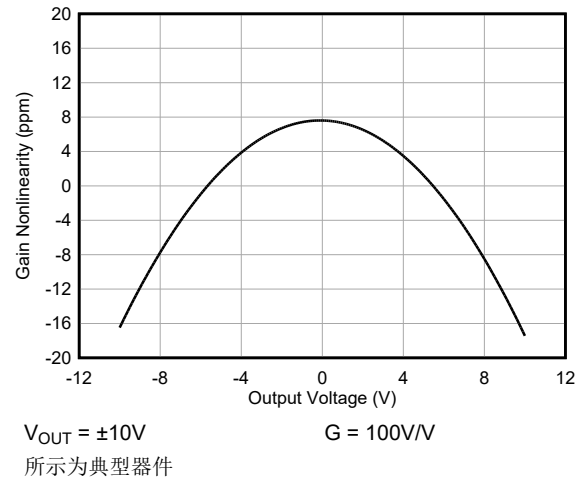
图 6-38. 增益非线性
