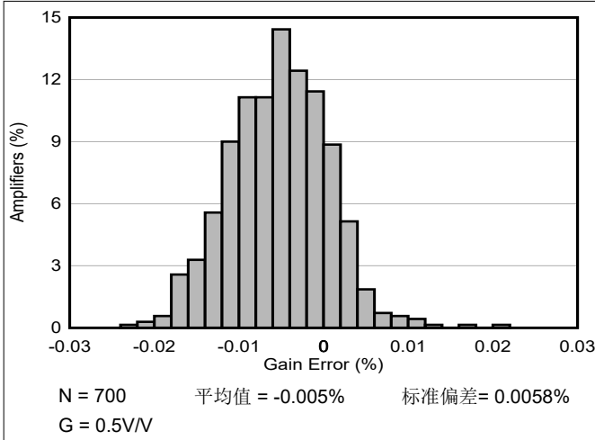
图 6-35. 增益误差的分布
