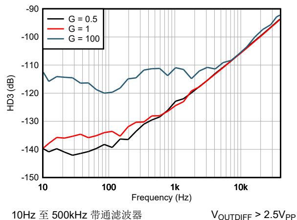
图 6-54. 三次谐波失真与频率间的关系
