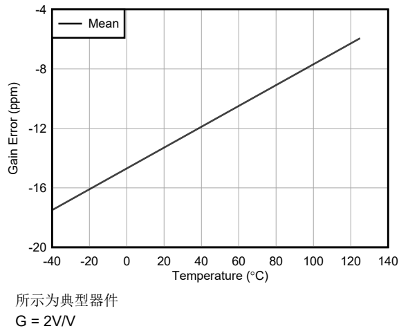
图 6-37. 增益误差与温度间的关系
