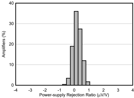
图 6-11. PSRR 分布
