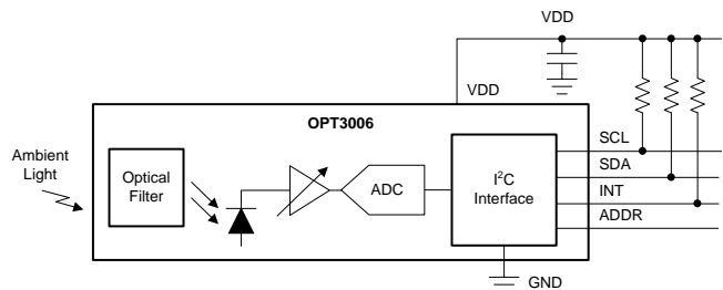
方框图
