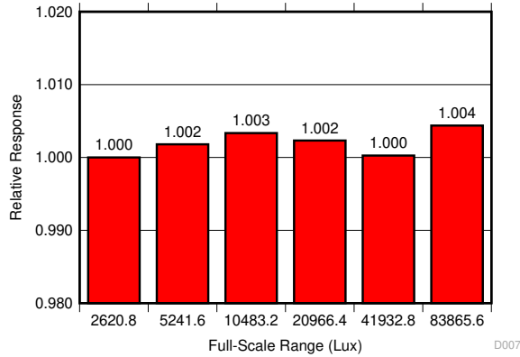
图 5-8. 满标量程匹配 (最高的 6 个量程)
