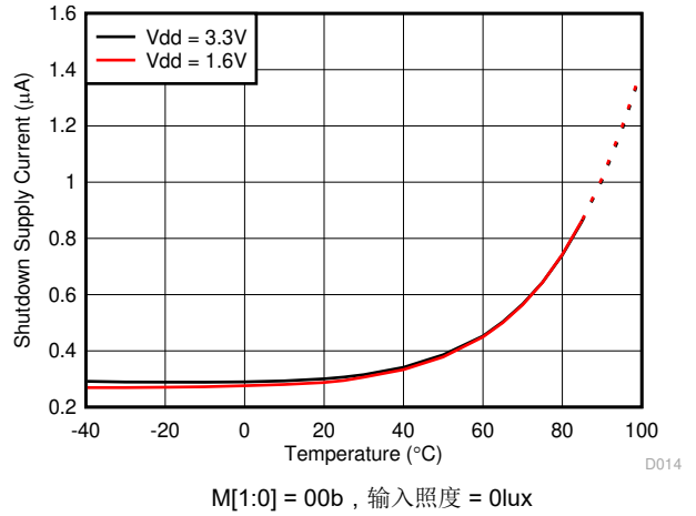
图 5-21. 关断电流与温度间的关系 ( 3 级 )
