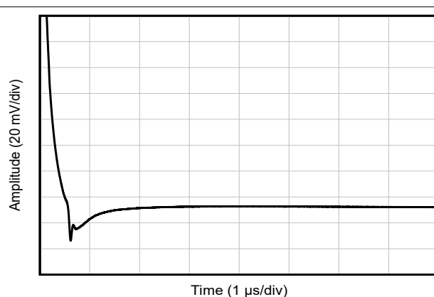
图 5-48. 稳定时间
