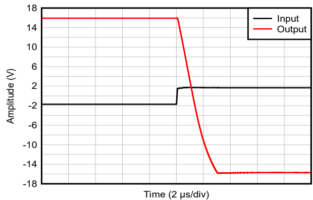
图 5-42. 正过负载恢复
