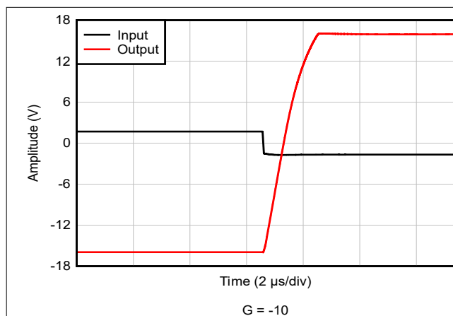
图 5-43. 负过载恢复
