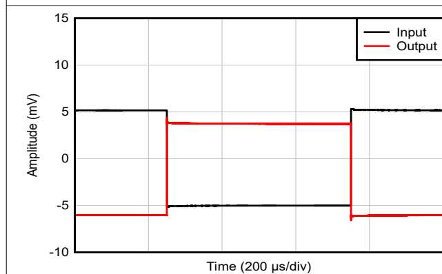
图 5-45. 小信号阶跃响应
