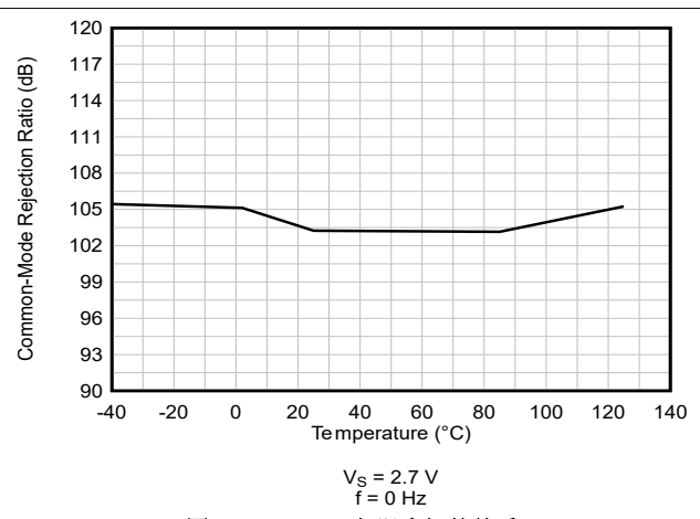
图 5-24. CMRR 与温度间的关系
