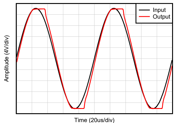
图 7-9. 无相位反转
