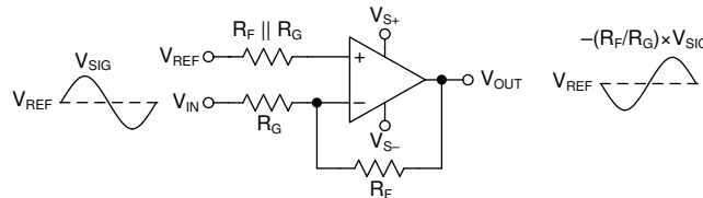
图 8-2. 反相放大器
