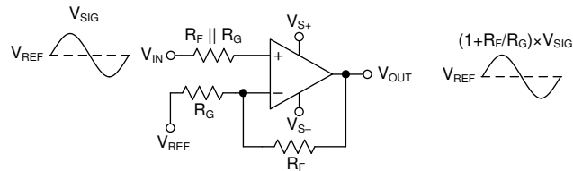
图 8-1. 同相放大器
