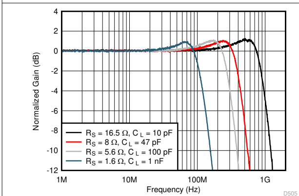
图 6-3. 微小信号频率响应与输出负载间的关系
