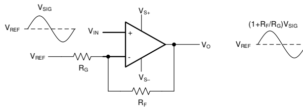
图 8-1. Noninverting Amplifier
