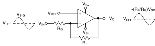
图 8-4. Inverting Amplifier
