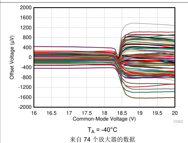
图 5-10. 失调电压与共模电压间的关系 (切换区域)
