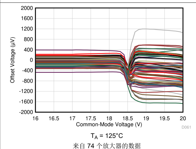
图 5-8. 失调电压与共模电压间的关系 (切换区域)
