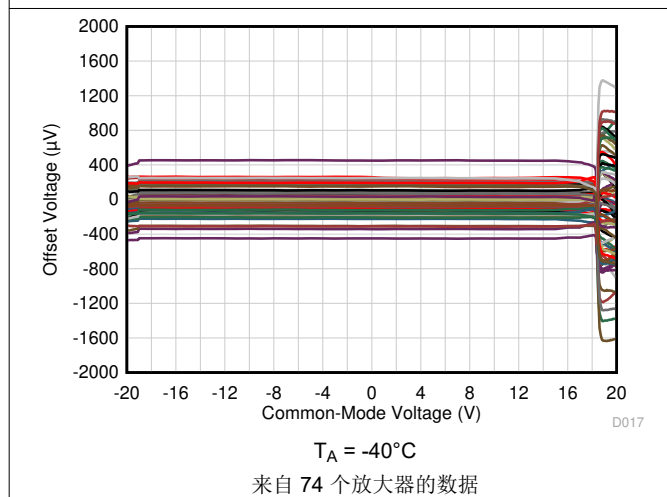
图 5-9. 失调电压与共模电压间的关系
