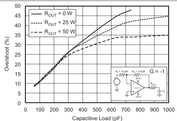
图 7-3. 小信号过冲与容性负载间的关系 (100mV 输出阶跃)
