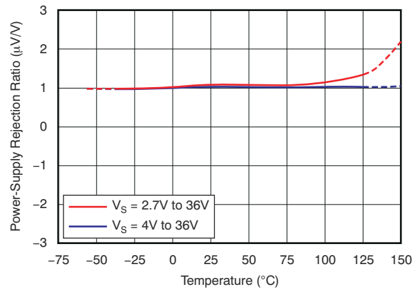
图 6-12. PSRR 与温度间的关系
