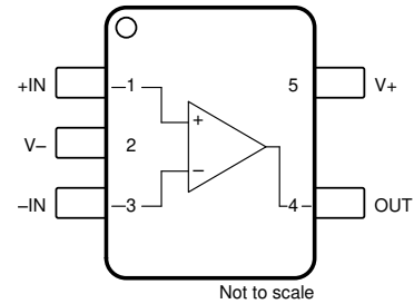
图 4-2. OPA397 DCK 封装 5 引脚 SC70 (顶视图)
