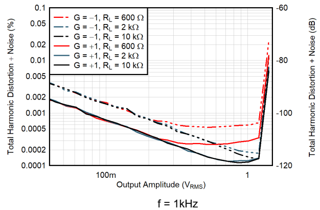
图 5-18. THD+N 与输出幅度间的关系
