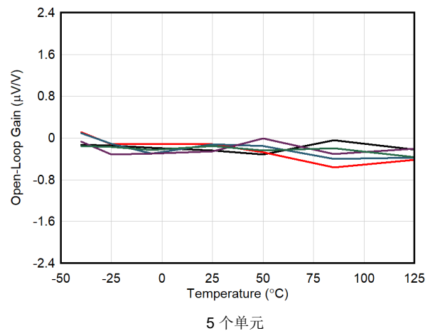
图 5-22. 开环增益与温度间的关系
