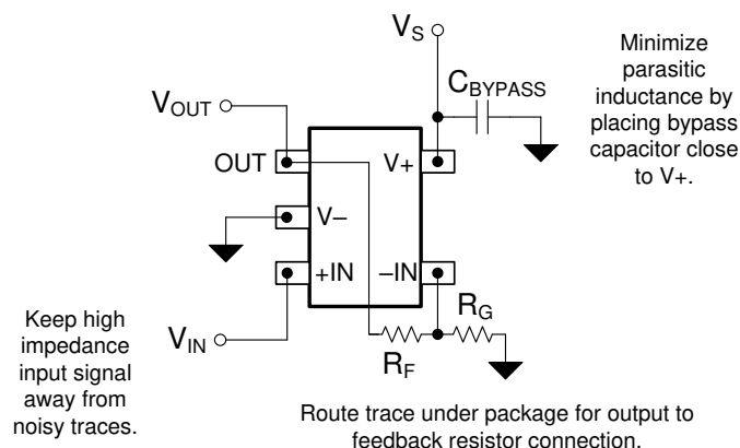
图 7-4. OPA397 布局示例
