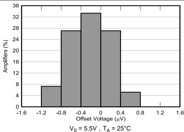
图 5-1. 失调电压分布图
