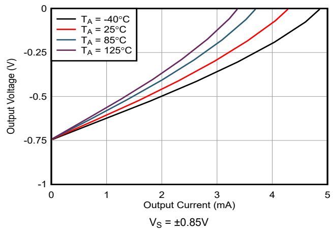
图 5-28. 输出电压与输出电流 (灌电流) 间的关系
