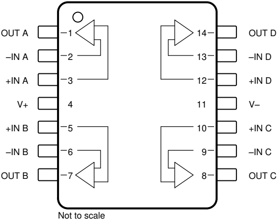
图 4-5. OPA4383：PW ( 预发布 ) 封装，14 引脚 TSSOP ( 顶视图 )
