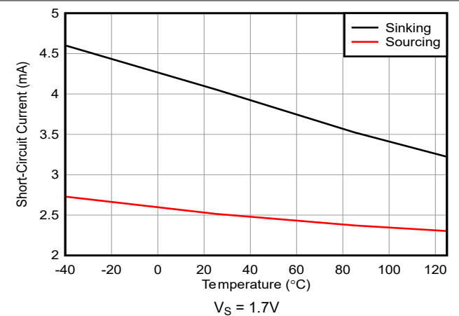
图 5-30. 短路电流与温度间的关系
