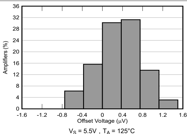
图 5-3. 失调电压分布图
