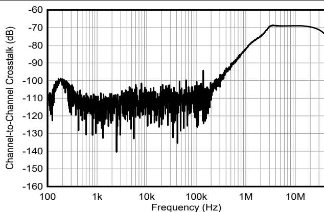
图 5-19. 通道间串扰
