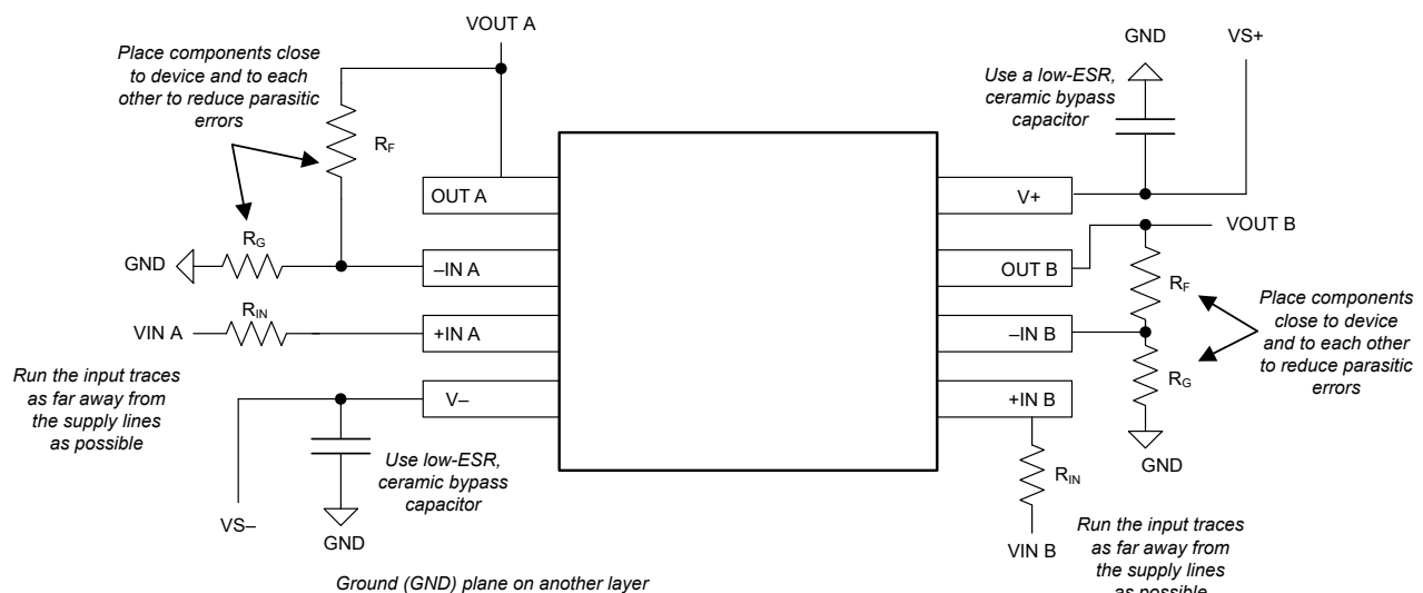
图 7-5. 布局示例
