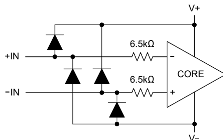
图 6-1. 等效输入电路
