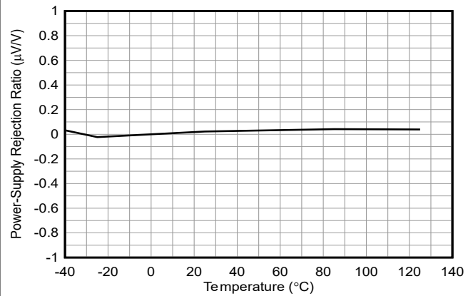
图 5-14. PSRR 与温度间的关系
