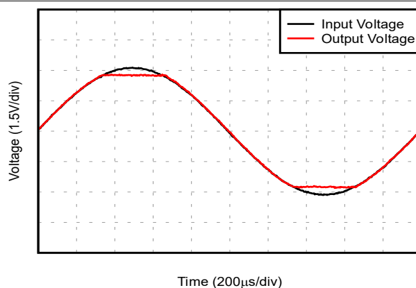
图 5-20. 无相位反转
