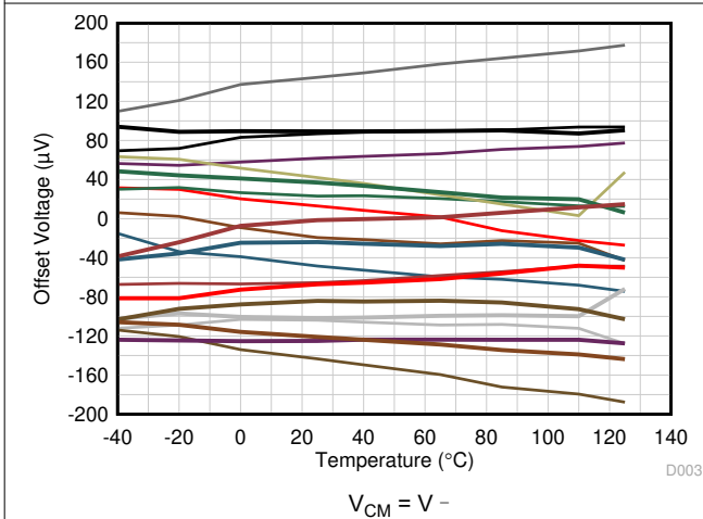
图 7-41. Offset Voltage vs Temperature (PMOS Input Pair)
