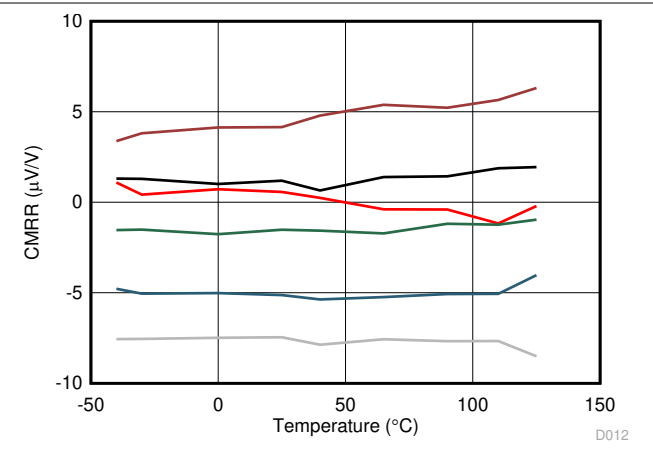
图 7-14. CMRR vs Temperature
