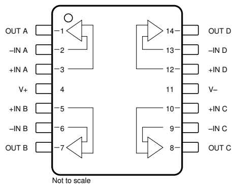
图 4-6. OPA4328 PW 封装 14 引脚 TSSOP ( 顶视图 )
