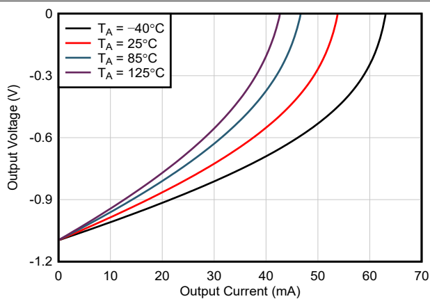
图 5-20. 输出电压摆幅与输出电流间的关系
