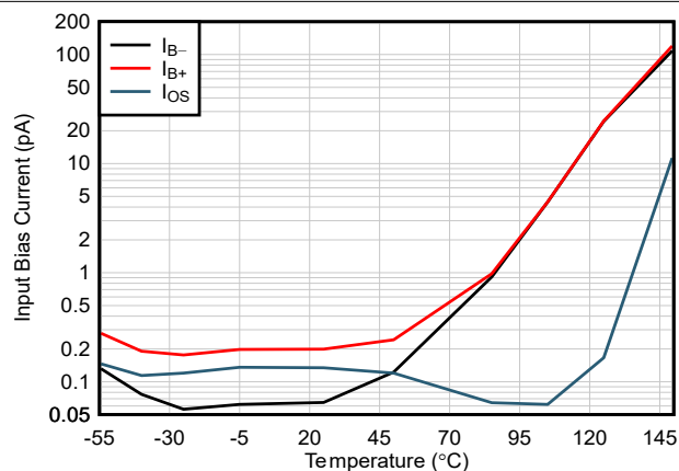
图 5-8. 输入偏置电流与温度间的关系
