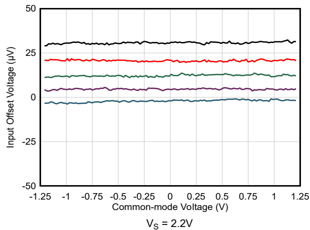
图 5-3. 失调电压与共模电压间的关系
