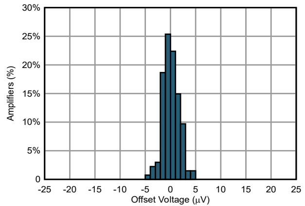
图 5-2. 失调电压产生分布
