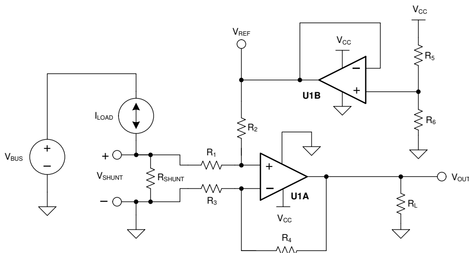
图 7-2. 双向电流感应原理图
