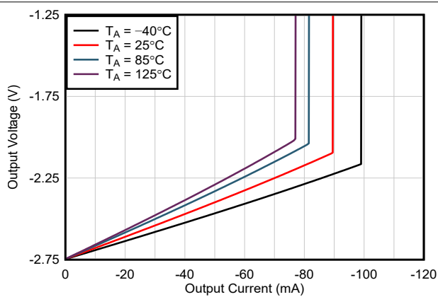
图 5-20. 输出电压摆幅与输出电流间的关系
