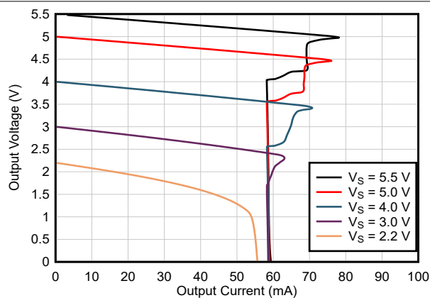
图 5-21. 输出电压摆幅与输出电流间的关系
