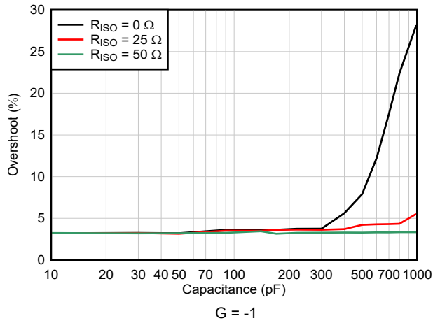
图 5-27. 小信号过冲与负载电容间的关系
