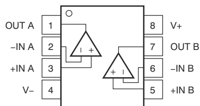
图 4-3. OPA2328 D 和 DGK 封装 8 引脚 SOIC 和 VSSOP (顶视图)
