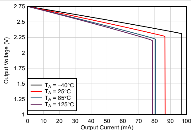
图 5-19. 输出电压摆幅与输出电流间的关系
