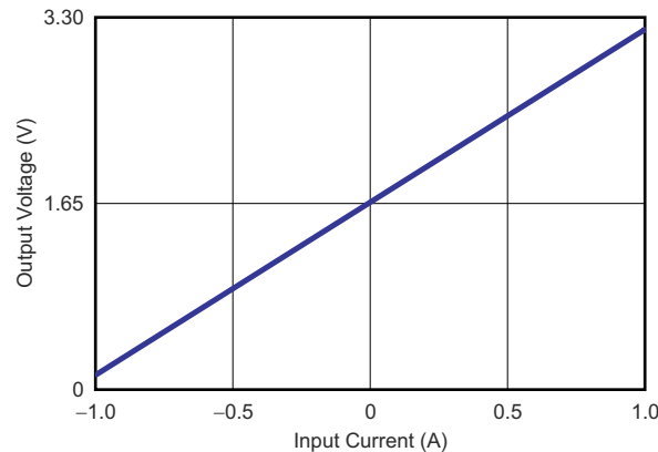
图 7-3. 双向电流检测电路性能：输出电压与输入电流间的关系
