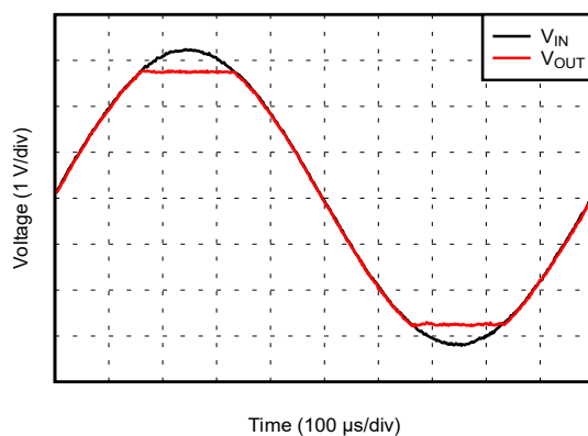
图 6-2. 无相位反转
