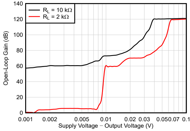
图 5-25. 开环增益与电源电压和输出电压差值间的关系
