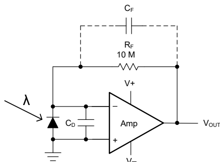
图 7-4. 双电源跨阻放大器
