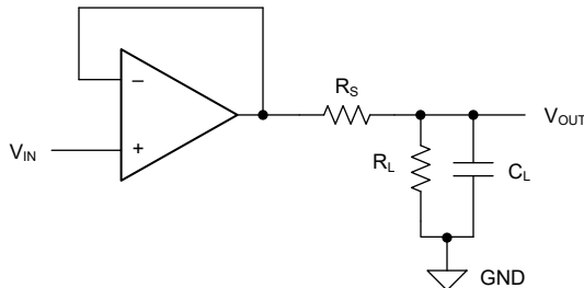
图 7-1. 增强容性负载驱动能力
