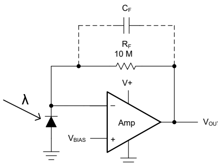
图 7-5. 单电源跨阻放大器
