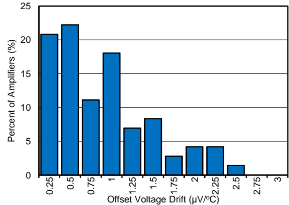
Figure 6. 偏移电压漂移分布
