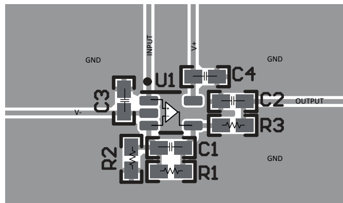
图 7-4. 同相配置的运算放大器电路板布局布线 - SC70 (DCK) 封装
