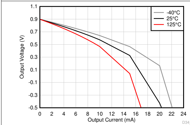
图 5-21. 输出电压摆幅与输出电流 (拉电流) 间的关系
