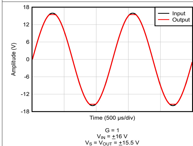
图 5-41. 无相位反转
