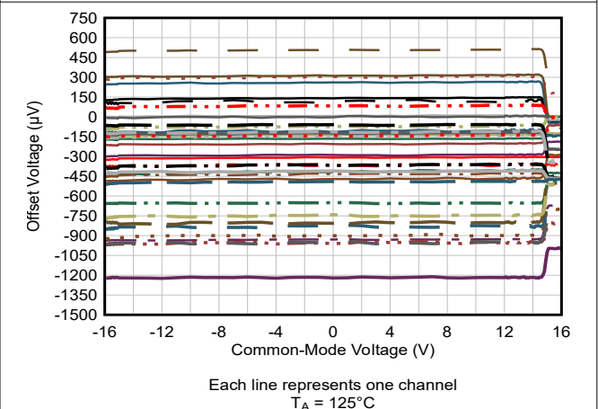
图 5-6. 失调电压与共模电压间的关系
