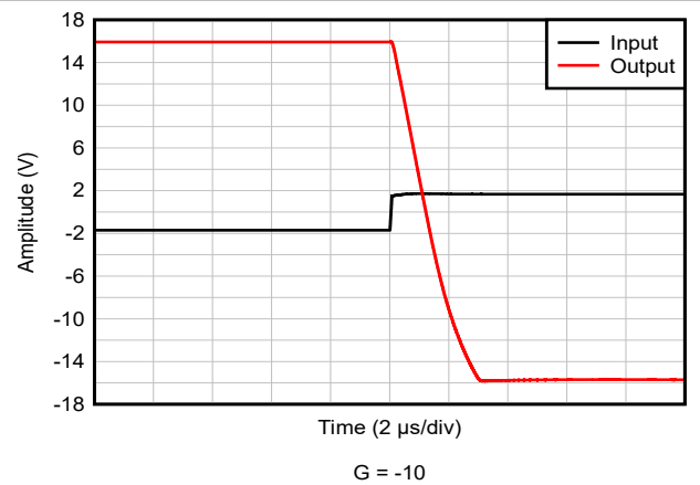
图 5-42. 正过载恢复
