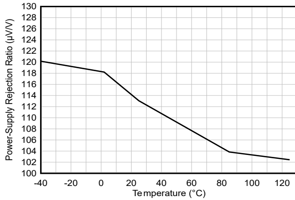
f = 0 Hz 图 5-25. PSRR 与温度间的关系
