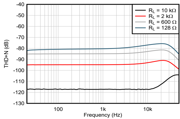
G = +1 V_{OUT} = 3 V_{RMS} BW = 80 kHz 图 5-28. THD+N 比与频率间的关系
