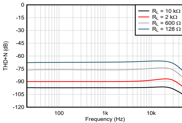
G = -1 V_{OUT} = 3 V_{RMS} BW = 80 kHz 图 5-29. THD+N 比与频率间的关系
