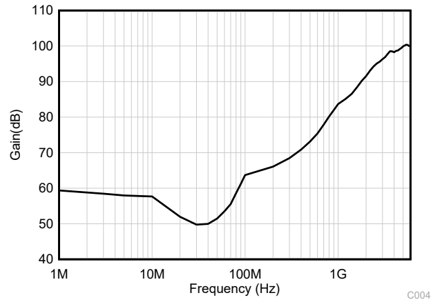
图 7-3. EMIRR 测试
