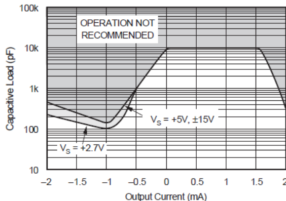
容性负载稳定性与输出电流间的关系
