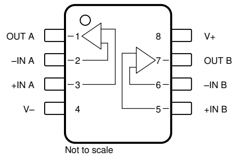
图 4-3. OPA2237 : D 封装，8 引脚 SOIC 和 DGK 封装，8 引脚 VSSOP (顶视图)
