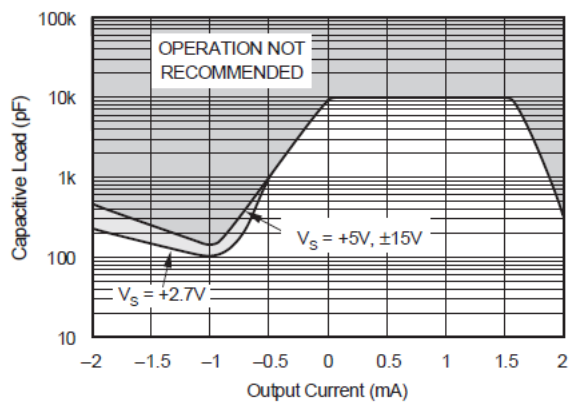
图 6-2. 容性负载稳定性与输出电流间的关系
