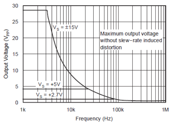
图 5-19. 最大输出电压与频率间的关系
