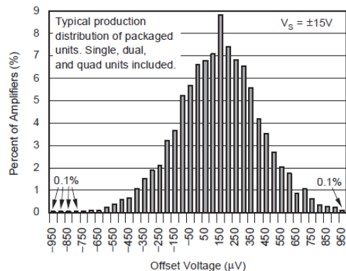
图 5-8. 失调电压产生分布
