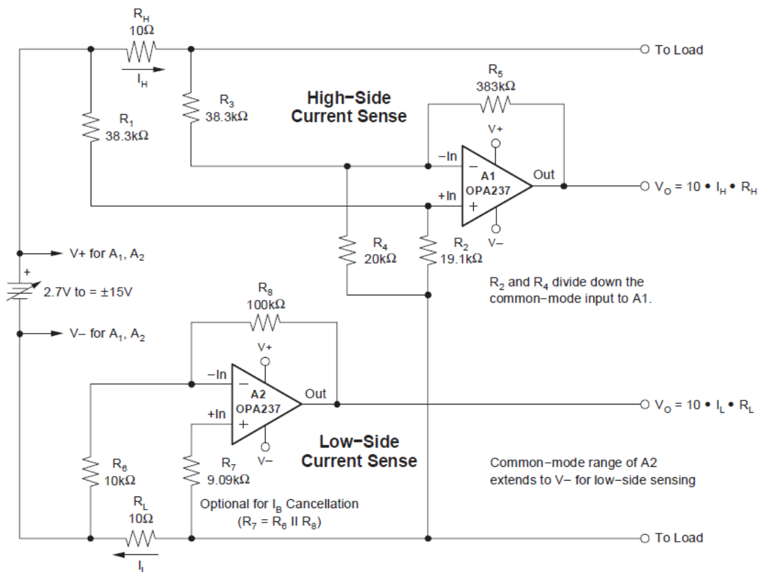
图 6-1. 低侧和高侧电池电流检测
