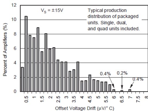
图 5-9. 偏移电压漂移产生分布
