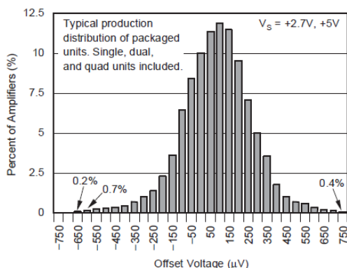
图 5-7. 失调电压产生分布
