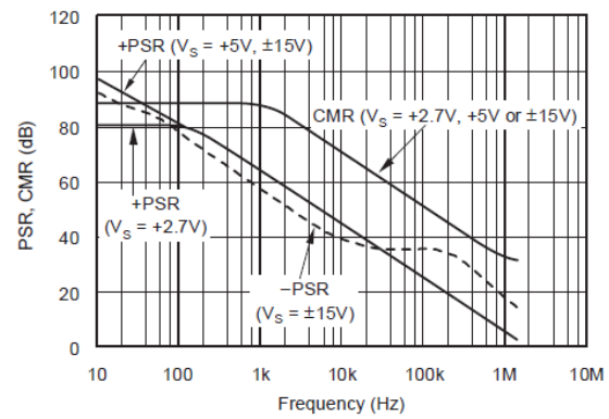
图 5-2. 电源和共模抑制与频率间的关系
