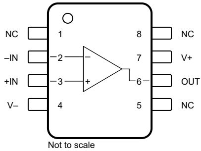
图 4-1. OPA237 : D 封装，8 引脚 SOIC (顶视图)
