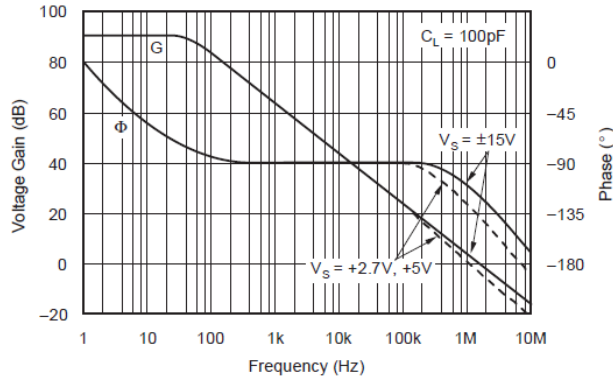
图 5-1. 开环增益和相位与频率间的关系
