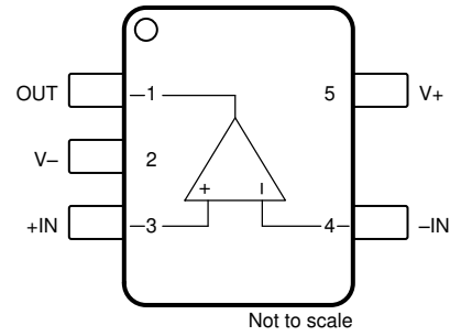
图 4-2. OPA237 : DBV 封装，5 引脚 SOT-23 (顶视图)
