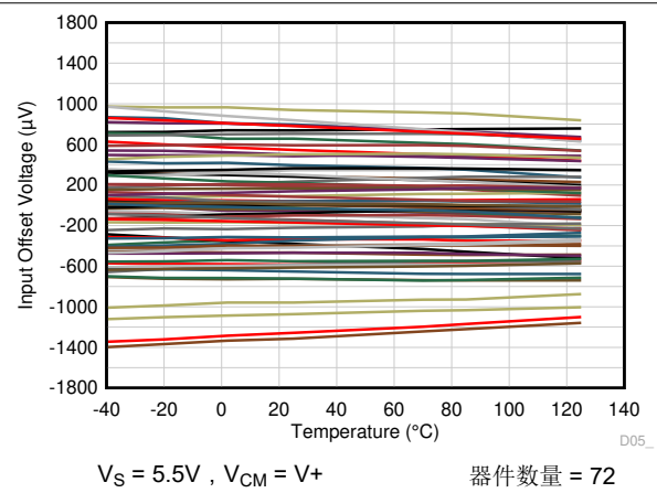
图 6-8. 输入失调电压与温度间的关系
