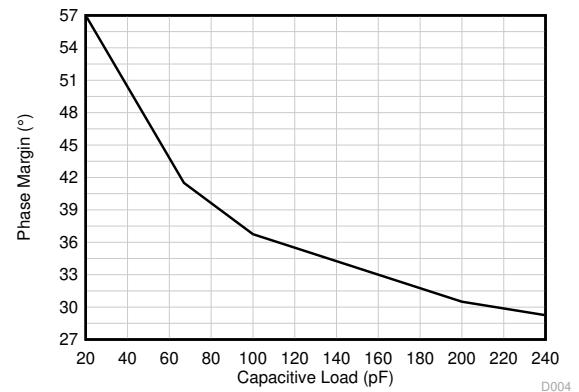
图 6-40. 相位裕度与容性负载间的关系
