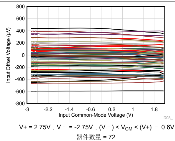
图 6-10. 失调电压与共模间的关系
