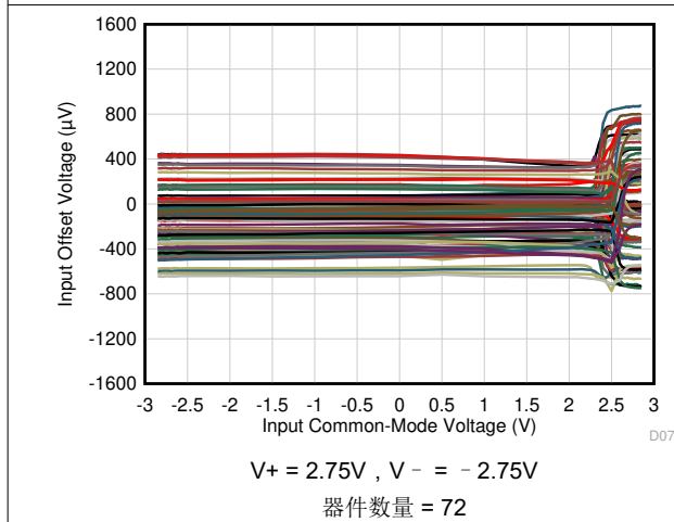
图 6-9. 失调电压与共模间的关系
