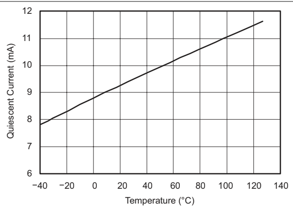
图 5-18. 静态电流与温度间的关系
