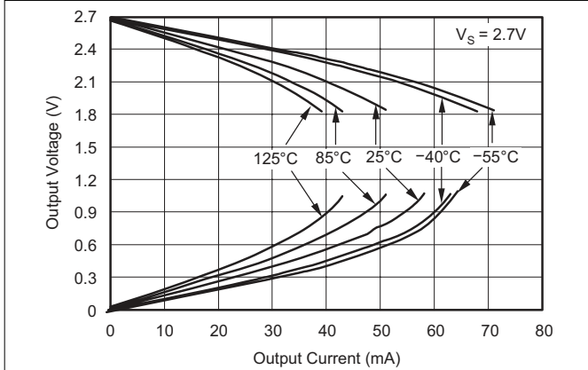
图 5-19. 输出电压摆幅与输出电流间的关系
