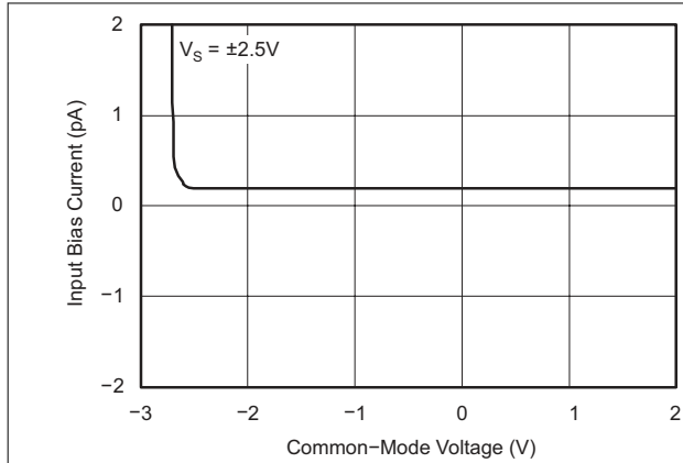
图 5-23. 输入偏置电流与共模电压间的关系
