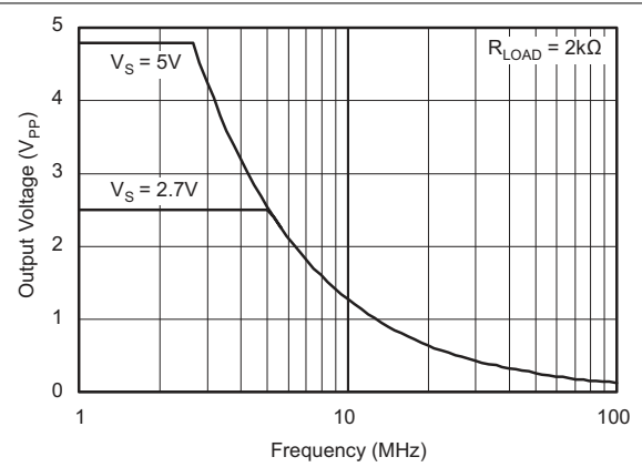
图 5-24. 最大输出电压与频率间的关系
