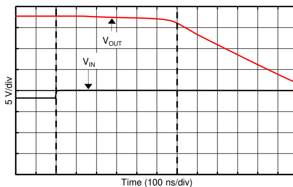
图 6-28. No Phase Reversal
