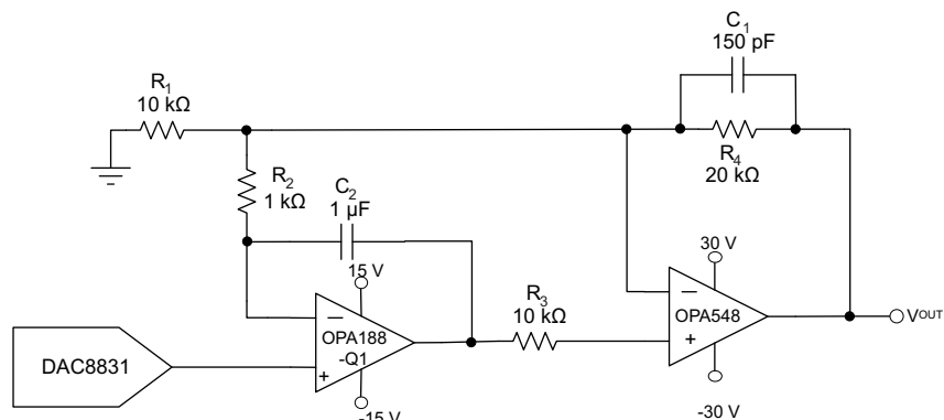
图 48. 可编程电源
