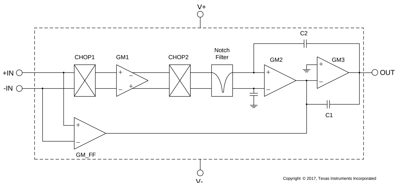
图 37. 功能框图
