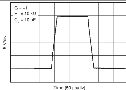
图 32. 大信号阶跃响应
