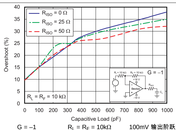
图 41. 小信号过冲与容性负载间的关系
