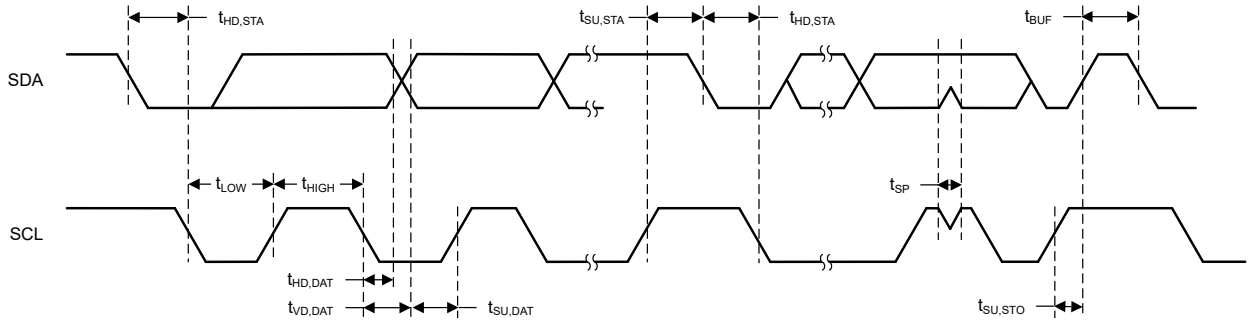
图 7-4. I2C 时序图
