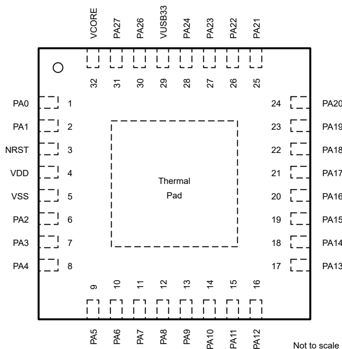
图 6-4. 32 引脚 RHB (0.5mm) (VQFN) 封装图
