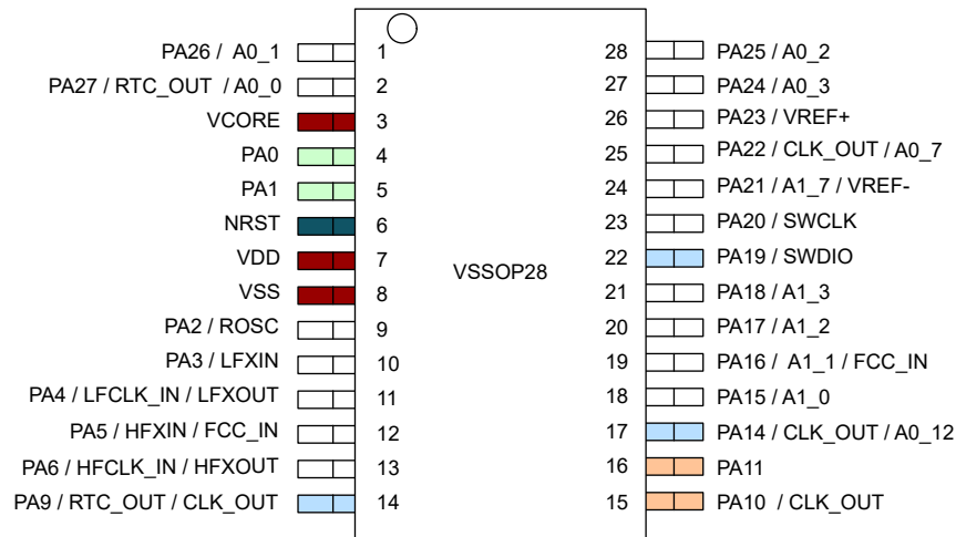
图 6-6. 28 引脚 DGS28 (VSSOP) (顶视图)
