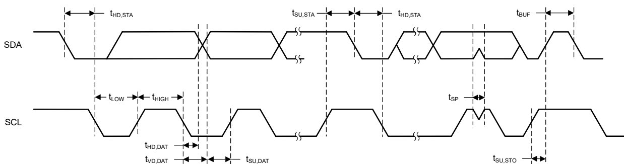
图 7-3. I2C 时序图
