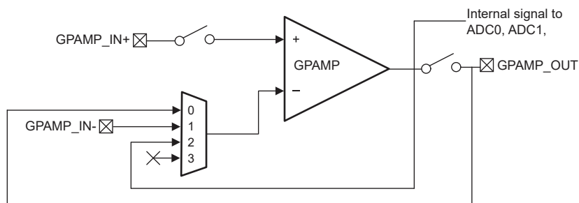
图 8-2. 模拟连接
