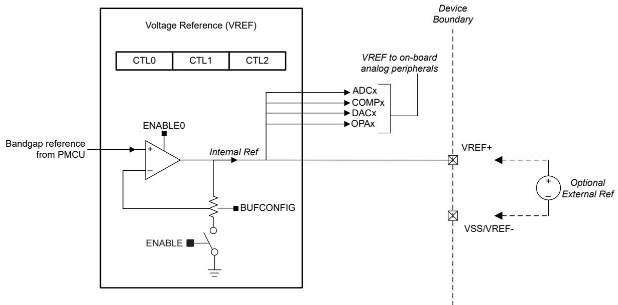
图 8-1. VREF 模块
