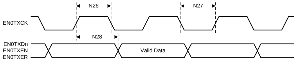
图 5-37. 100-Mbps MII Transmit Timing
