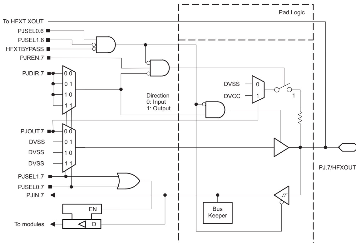
图 5-16. Port PJ (PJ.7) Diagram
