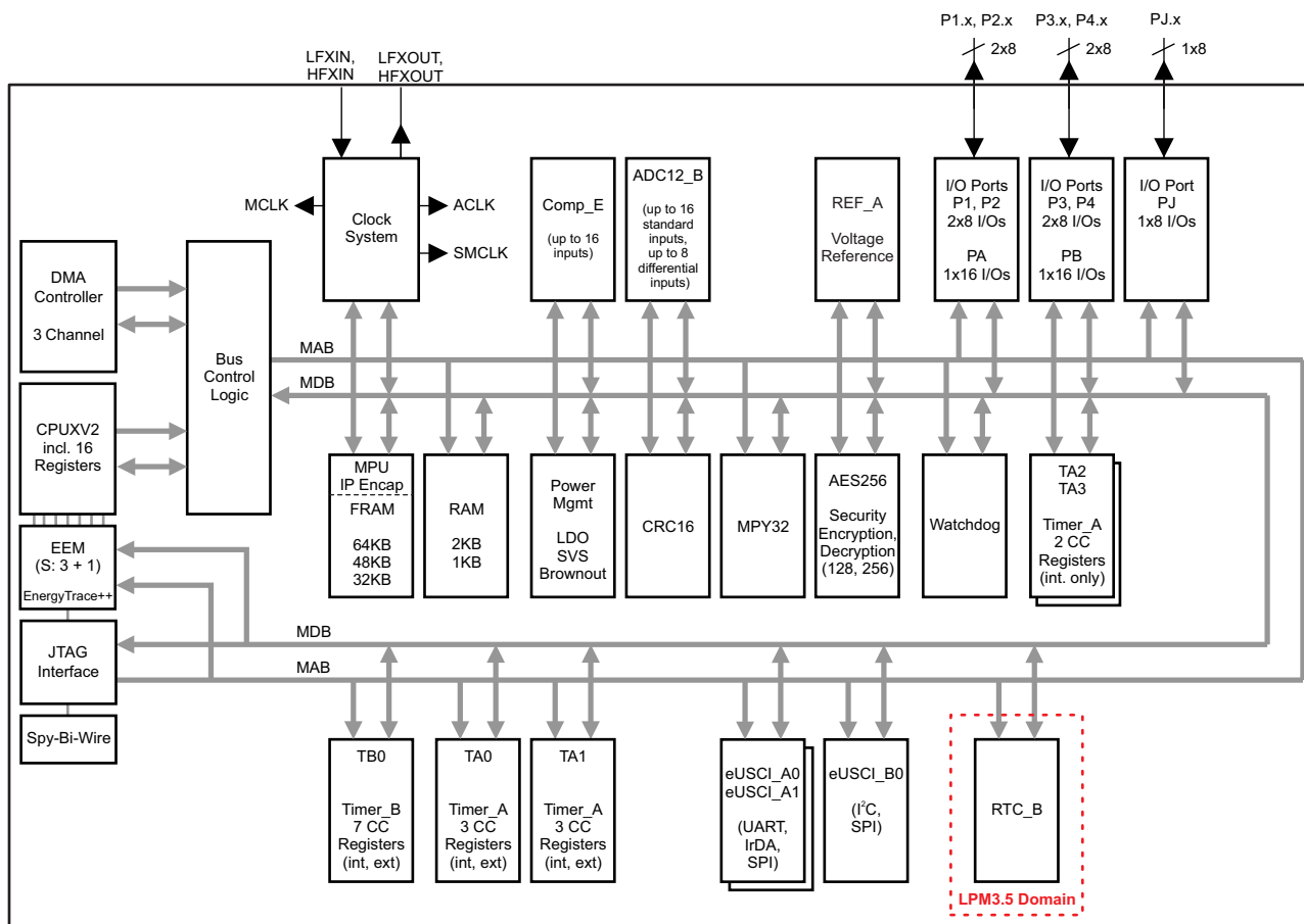
图 1-1. 功能方框图
