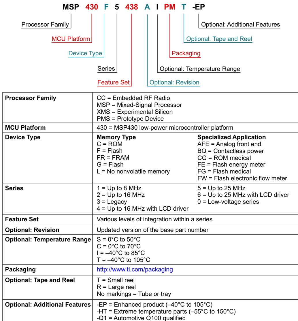
图 11-1. Device Nomenclature
