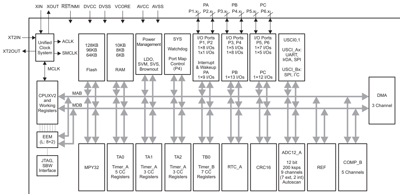
图 1-1. MSP430F534x 方框图
