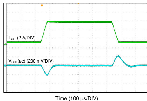
图 7-5. DCM 模式
