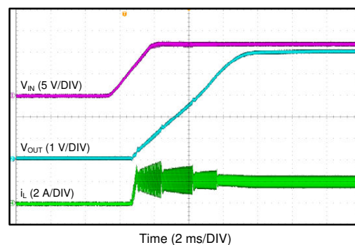
图 7-3. 由 VIN 启动
