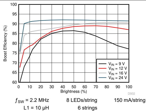
图 6-3. Boost Efficiency
