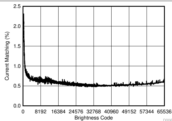
图 6-7. Current Matching
