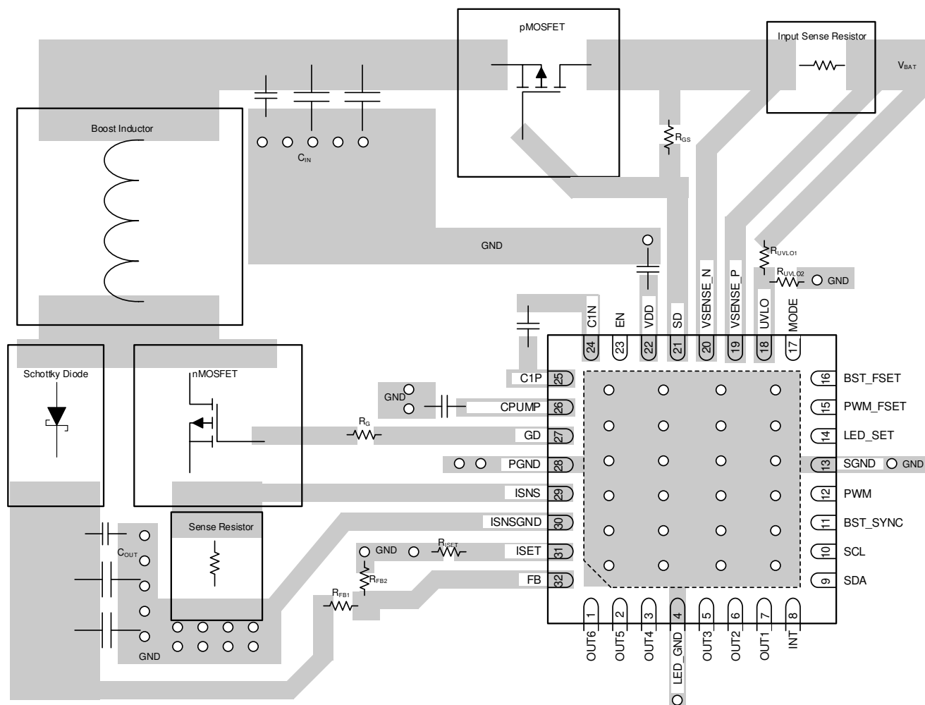
图 10-1. LP8866S-Q1 Layout Guidelines
