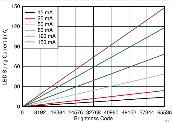
图 6-6. Current Linearity
