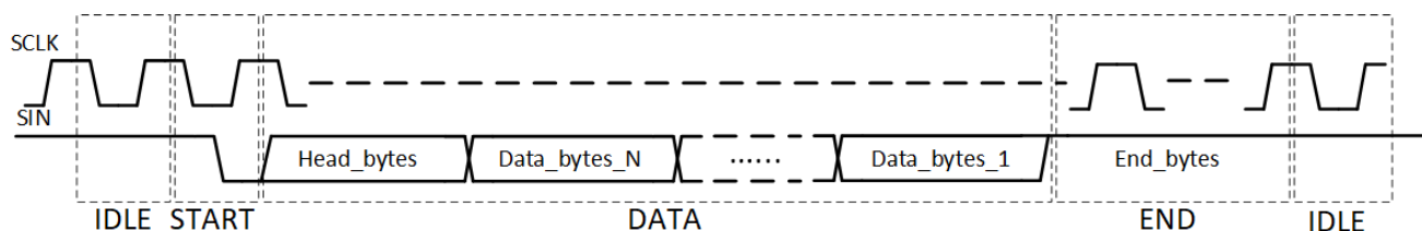
图 8-17. CCSI Frame
