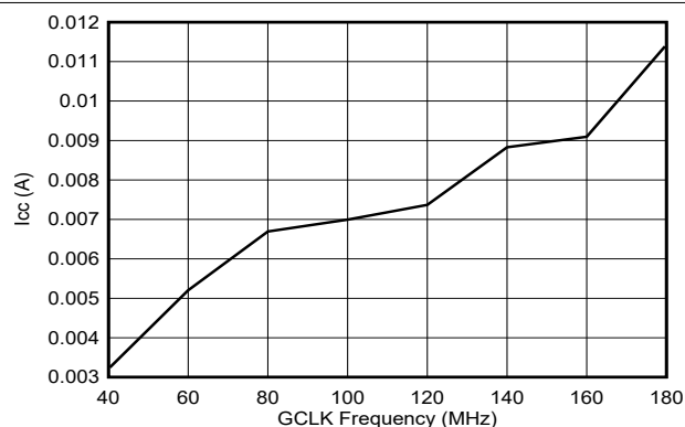
图 7-7. Icc Current vs GCLK Frequency
