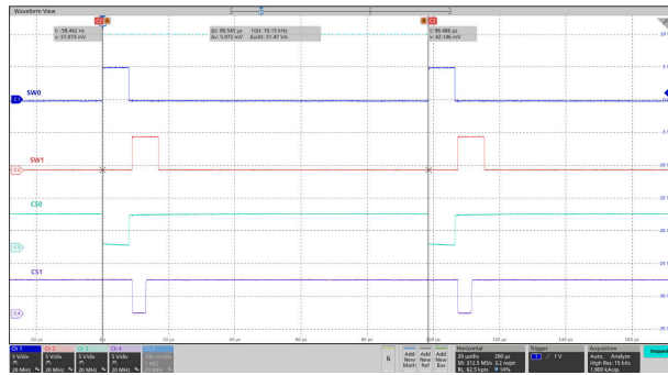
图 9-3. SW0、SW1、CSR0(CS0)、CSG0(CS1) 的扫描线和电流阱波形
