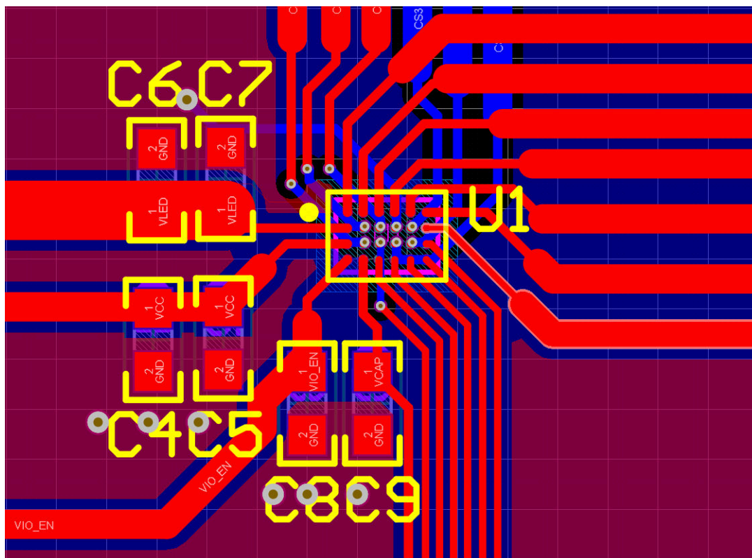
图 9-10. LP5867 布局示例
