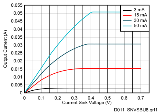
图 6-9. 电流阱电压与电流间的关系
