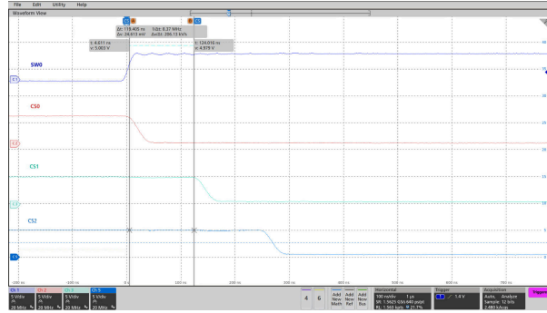
图 9-9. 已启用 PWM 相移
