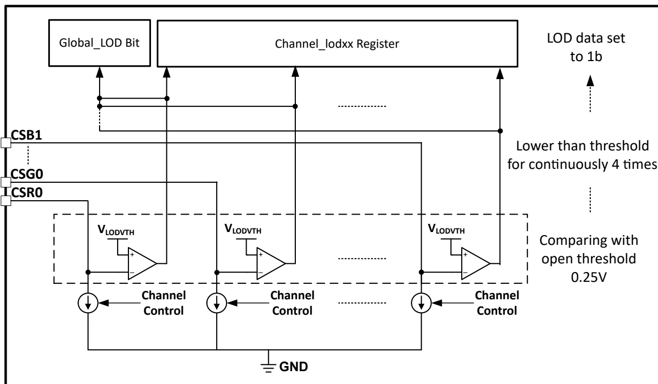
图 7-11. LOD 电路
