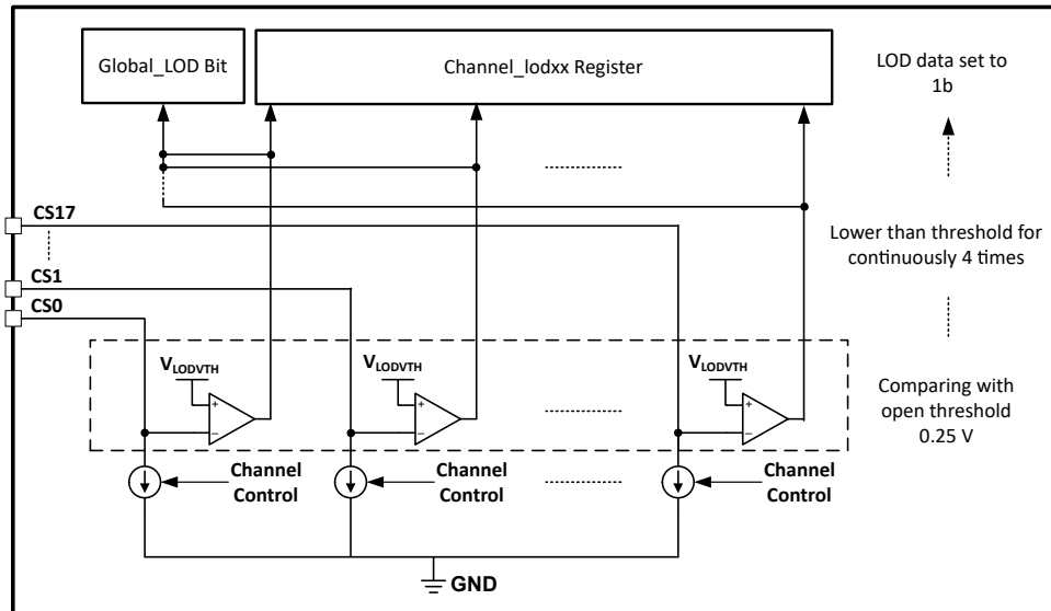
图 8-11. LOD Circuits
