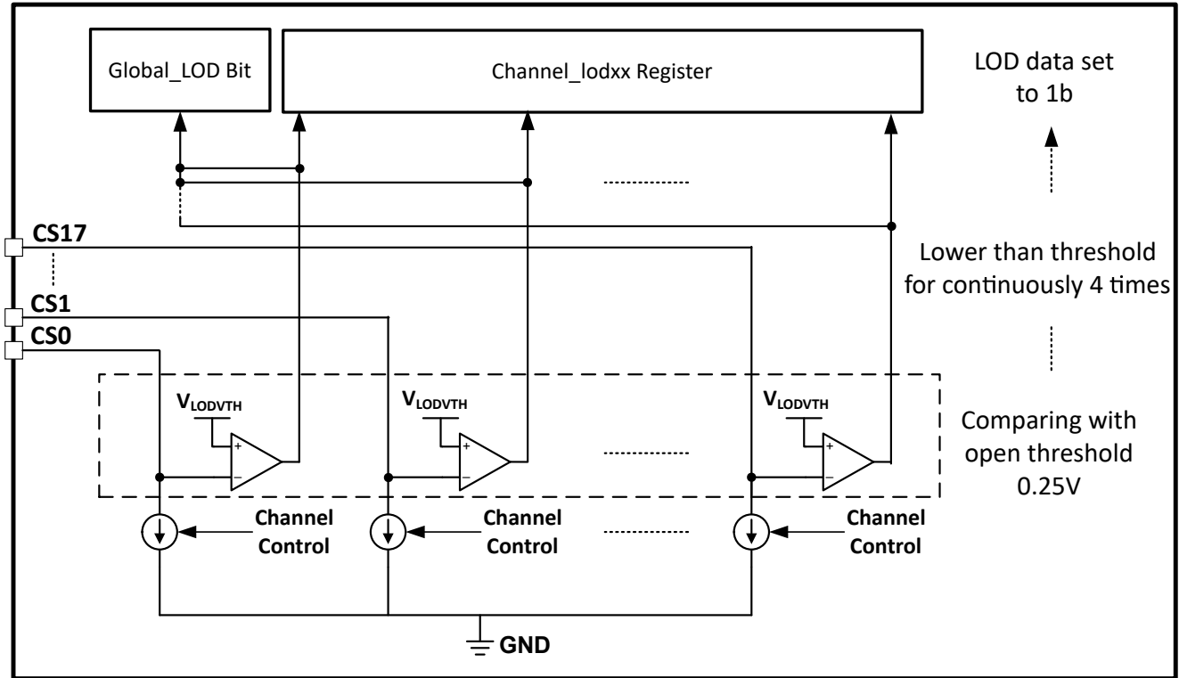
图 8-11. LOD Circuits
