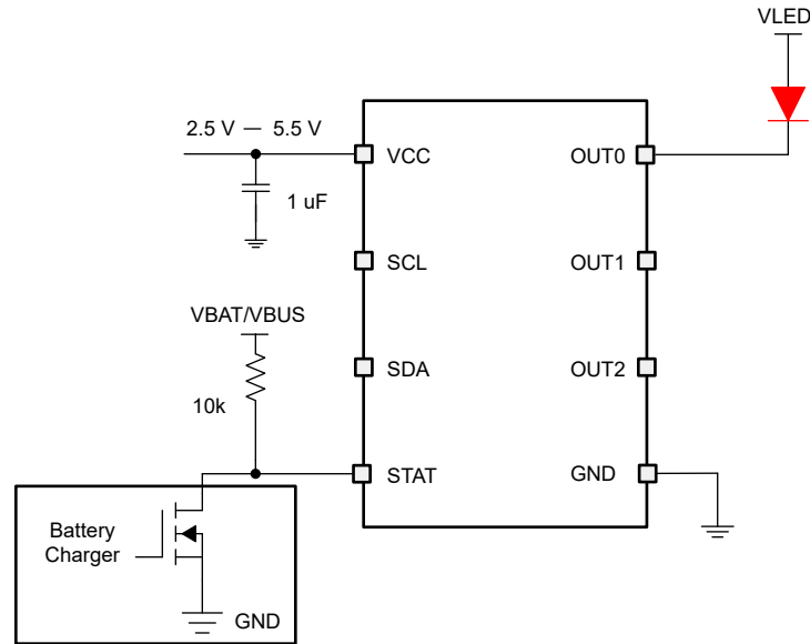
图 7-11. 即时闪烁应用电路
