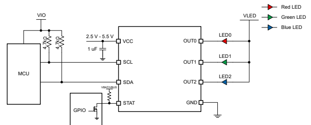
LP5815 简化原理图
