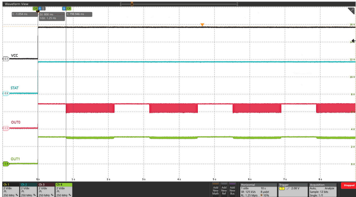
图 8-5. 上电即时闪烁波形
