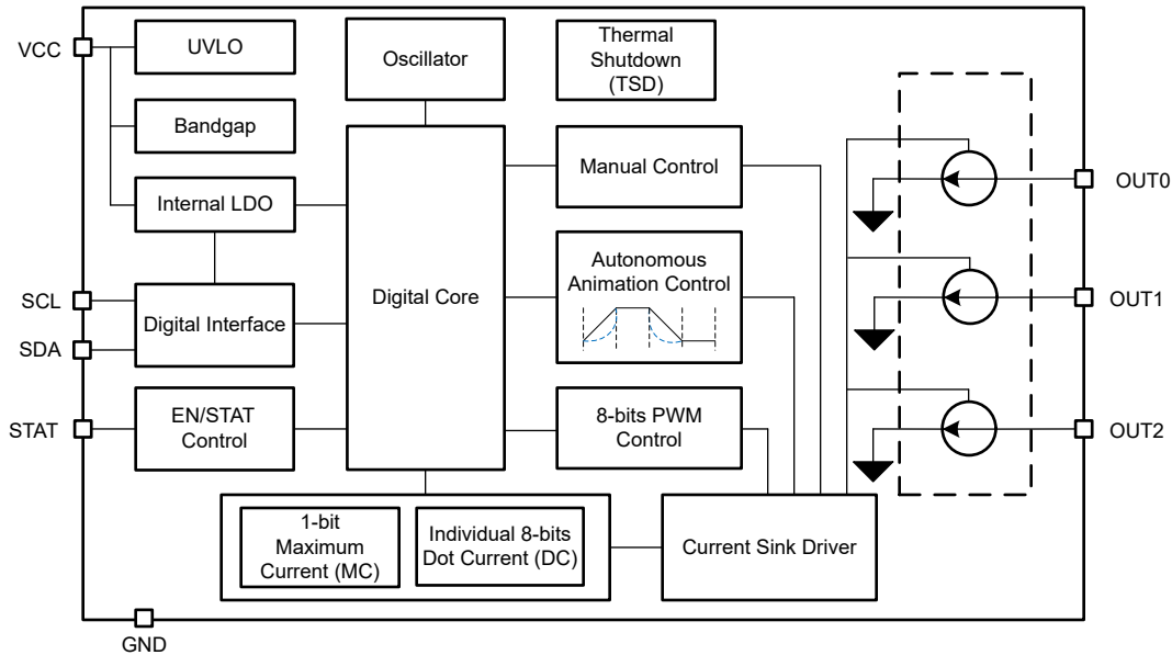
图 7-1. LP5815 功能模块
