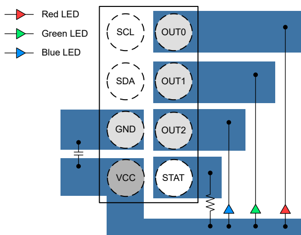
图 8-8. LP5815 YCH 封装布局示例
