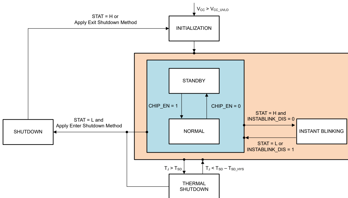
图 7-12. 功能模式
