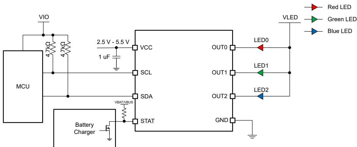
图 8-1. 典型应用 - LP5815 驱动 RGB LED
