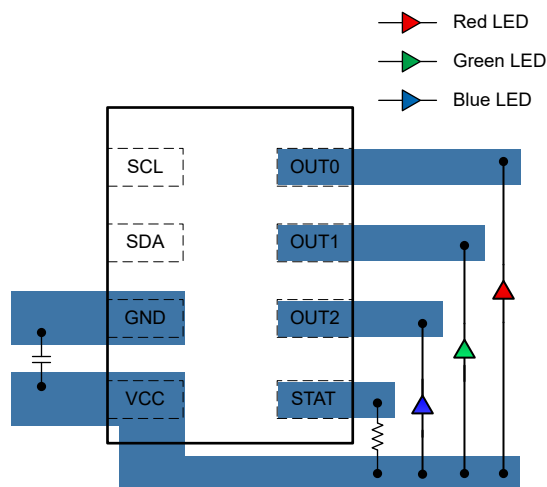
图 8-7. LP5815 DRL 封装布局示例
