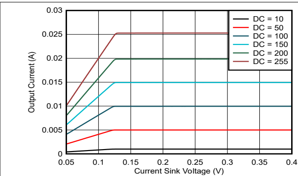
图 6-2. 电流阱电压与电流间的关系 ( MC = 0 ， V_{CC} = 2.5\text{V} )
