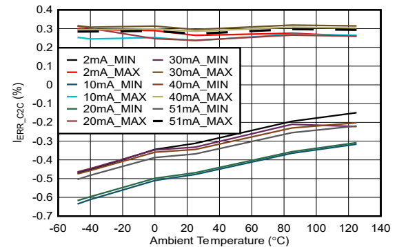
图 6-11. 通道间电流精度与温度间的关系 (MC = 1, VCC = 2.5V)
