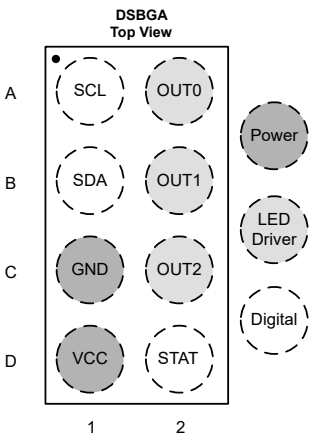
图 5-2. LP5815 YCH 封装 8 引脚 DSBGA 顶视图
