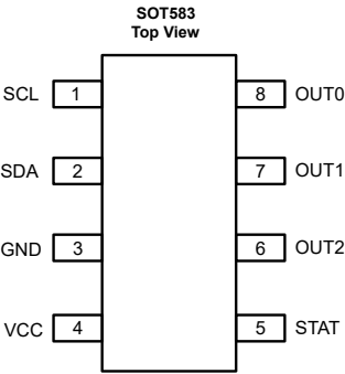
图 5-1. LP5815 DRL 封装 8 引脚 SOT583 顶视图
