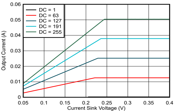
图 6-2. 电流阱电压与电流间的关系 (MC = 1)
