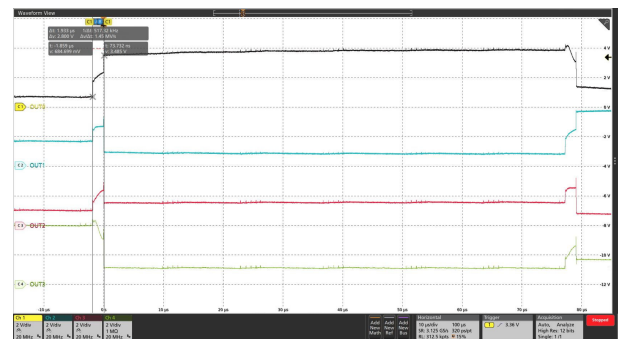
图 8-4. OUT0、OUT1、OUT2、OUT3 的扫描线路和电 流阱波形
