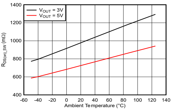
图 6-6. 扫描线开关 MOSFET R_{\text{DS(on)}}
