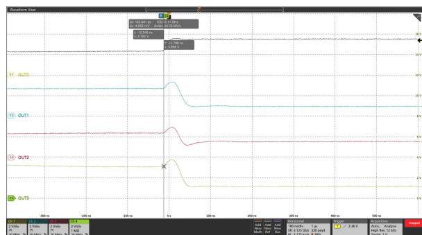
图 8-5. OUT0、OUT1、OUT2、OUT3 的扫描线路开关 波形
