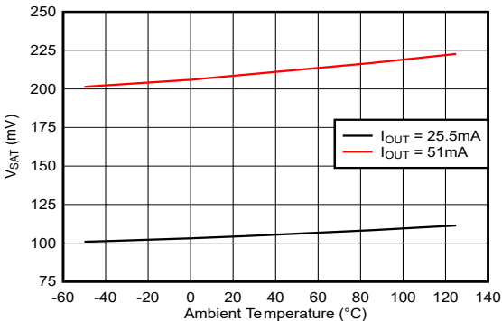
图 6-3. V_{\text{SAT}} 与温度间的关系
