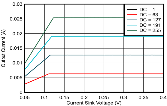
图 6-1. 电流阱电压与电流间的关系 (MC = 0)
