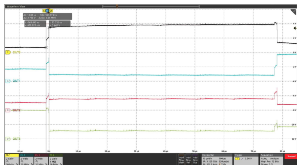
图 8-3. OUT0、OUT1、OUT2、OUT3 的扫描线路和电 流阱波形
