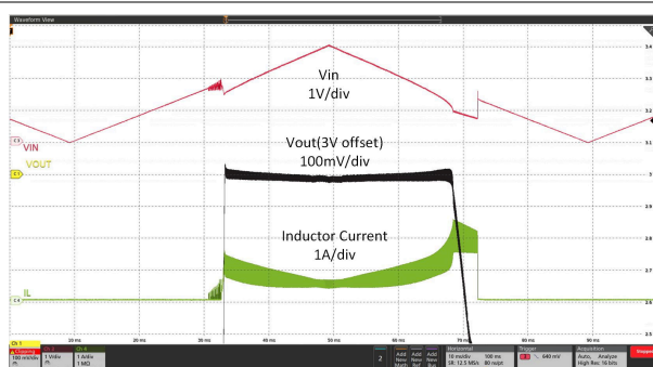
V_{IN} = 0V 至 3V 扫描, V_{OUT} = 3V , 6.6\Omega 电阻负载
